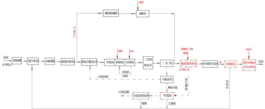
图4-1 江海污水处理厂废水处理工艺流程图
