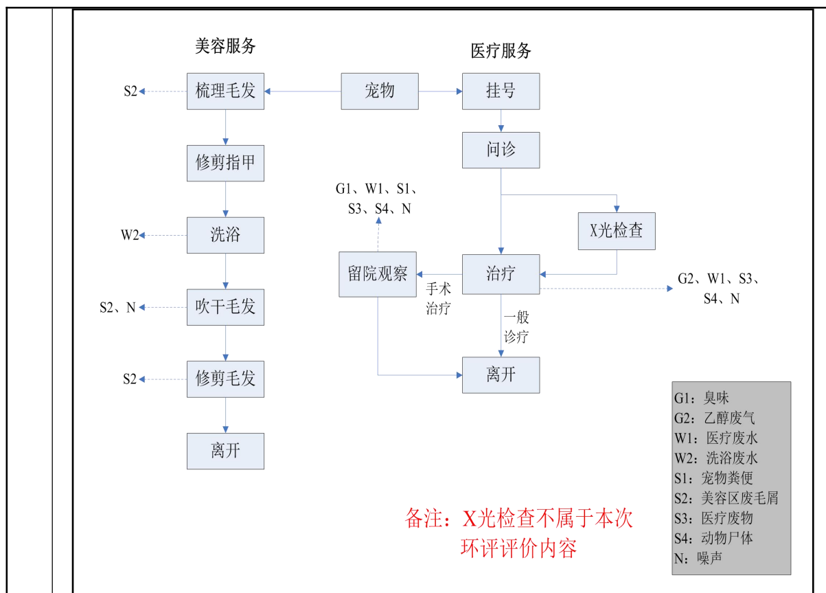
图 2.3 项目美容、医疗服务流程及产排污环节图
