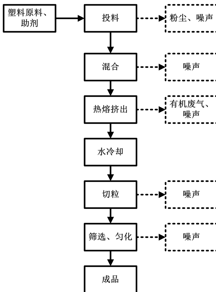
图2-1 项目生产工艺流程图
