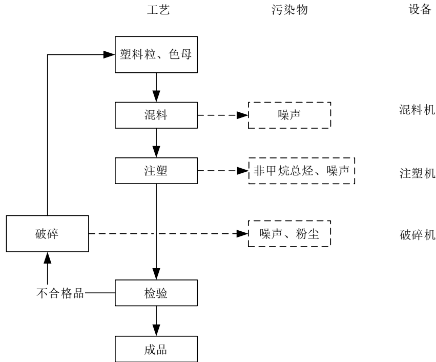
图 2-2 塑料配件生产工艺流程图
