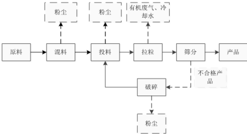
图 2-2 改性塑料生产工艺流程及产污环节示意图
