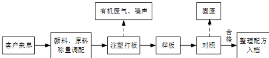
图 2-1 注塑打板工艺流程及产污环节示意图
