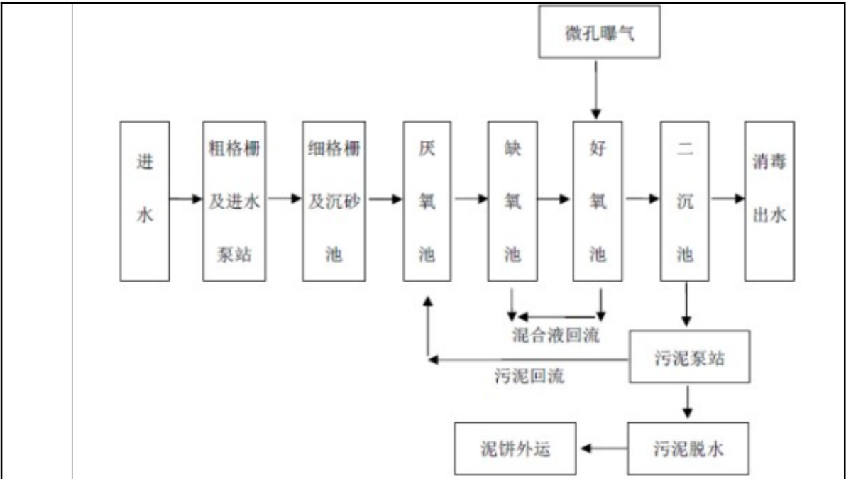
图 4-1 荷塘镇生活污水处理厂一、二期工程工艺流程图
