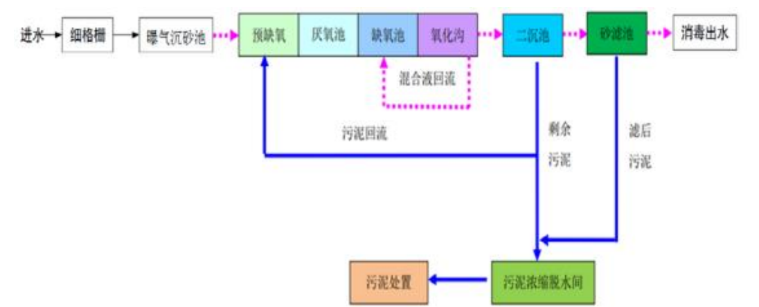
图 4-1 荷塘镇生活污水处理厂工艺流程图
