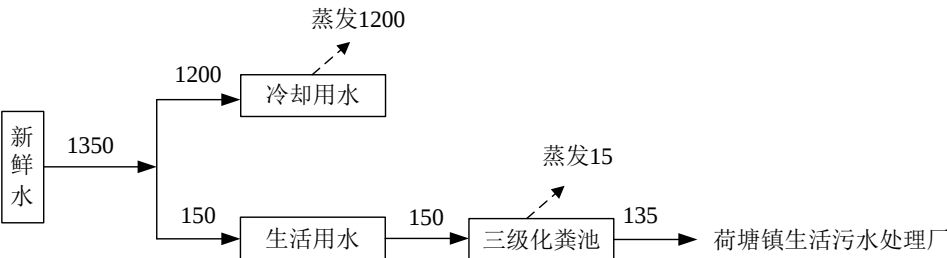
图 2-2 远期项目水平衡图（单位：m 3 /a）
