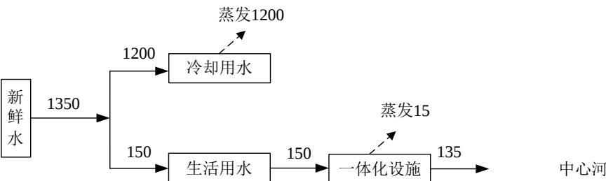
图 2-1 远期项目水平衡图（单位：m 3 /a）
