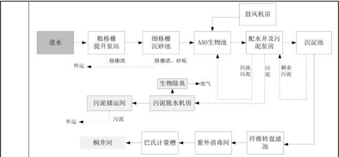
图 4-1 棠下污水处理厂污水处理工艺流程图
