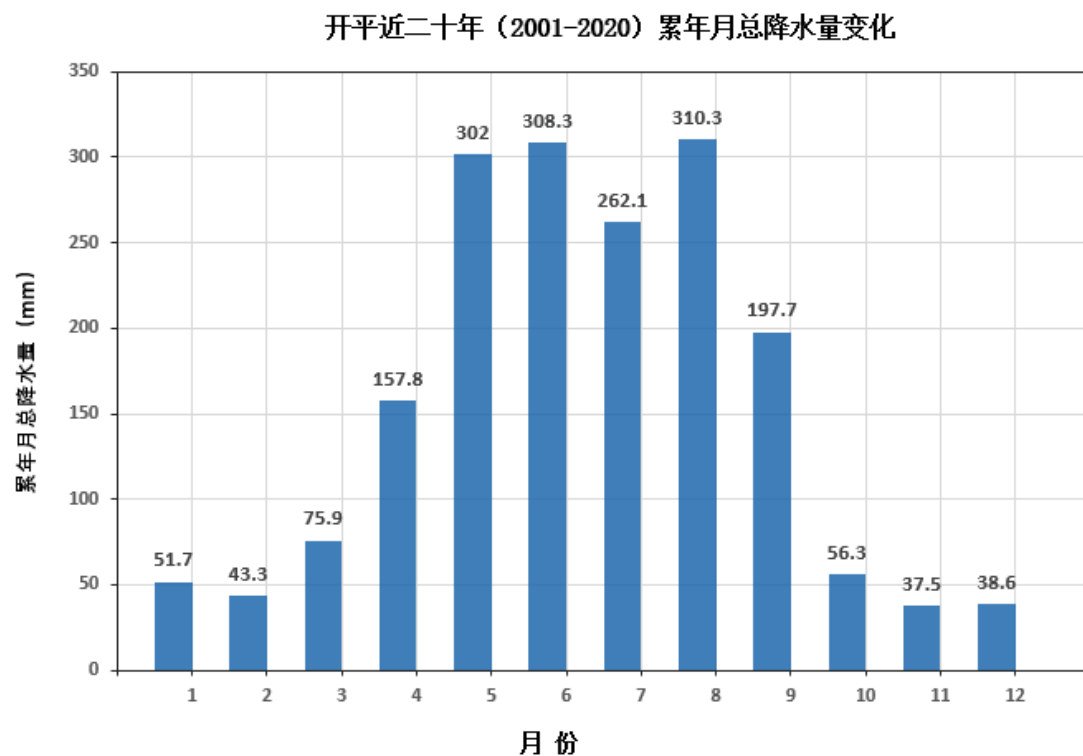
图 5.2.3-6 开平近 20 年月平均降水量（单位：毫米）
