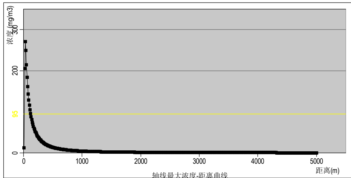
图 5.2.6-1 下风向不同距离处一氧化碳的最大浓度（最不利气象条件）
