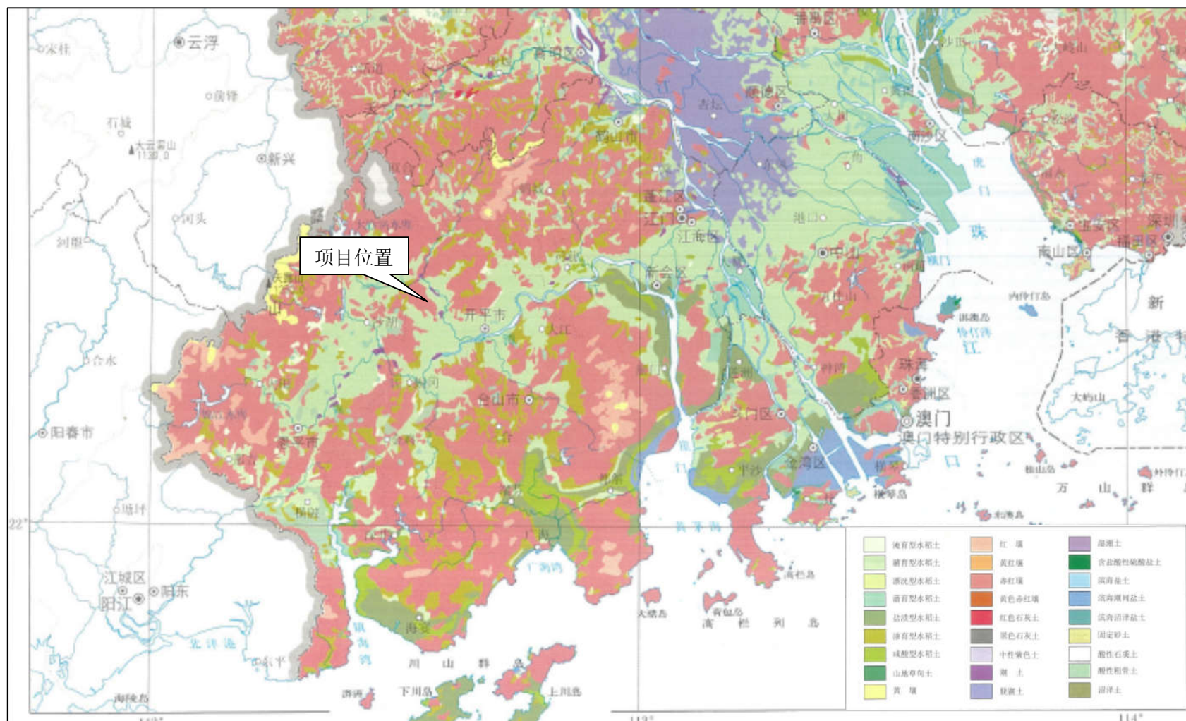
图 4.2.5-2 项目土壤类型图
