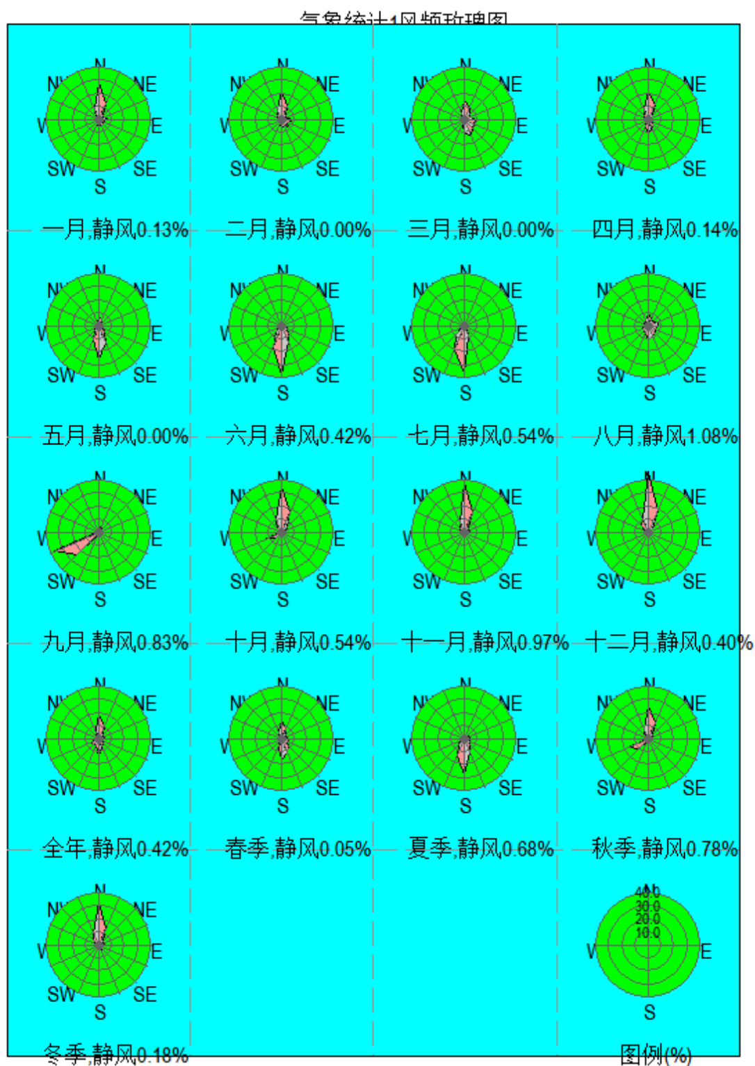
图5.2.3-15 开平2020年年风向频率玫瑰图
