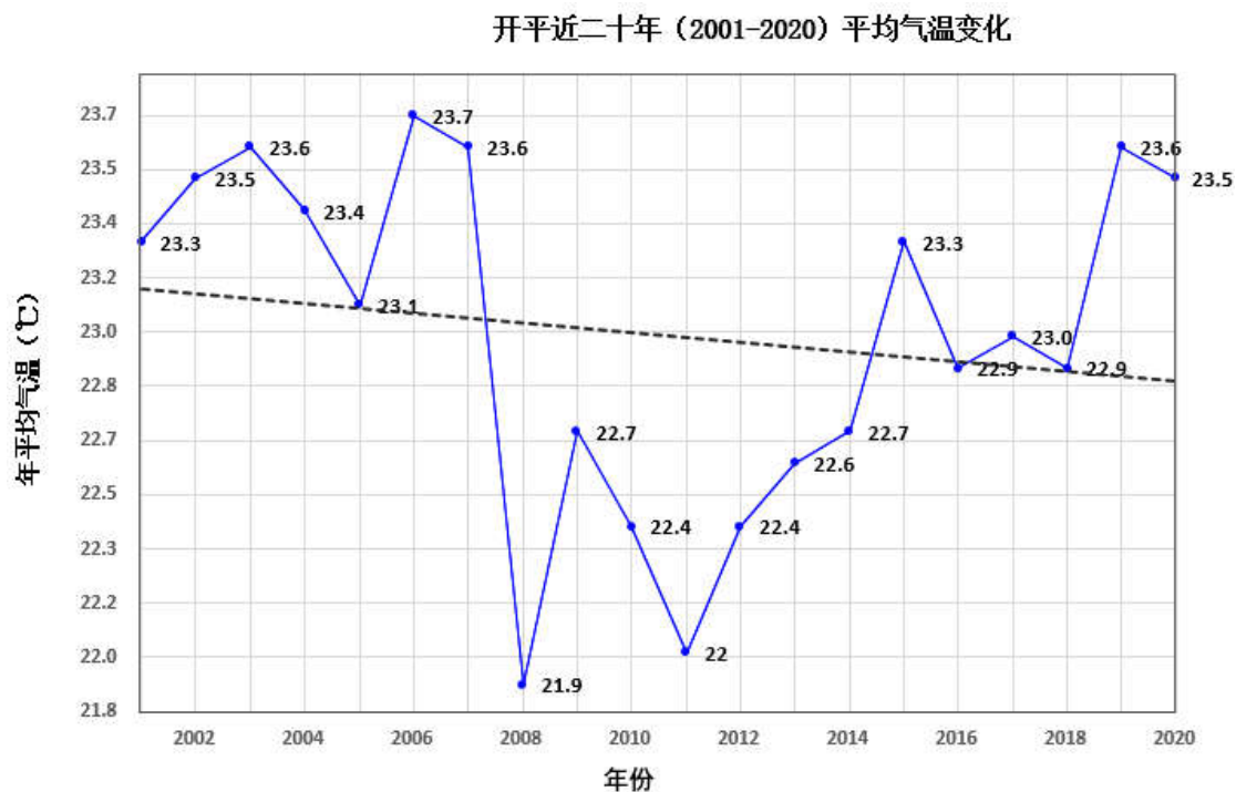
图 5.2.3-5 开平（2001-2020）年平均气温（单位：°C，虚线为趋势线）
