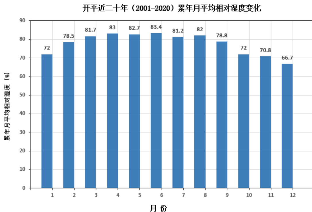
图 5.2.3-10 开平近 20 年月平均相对湿度统计结果（纵轴为百分比）
