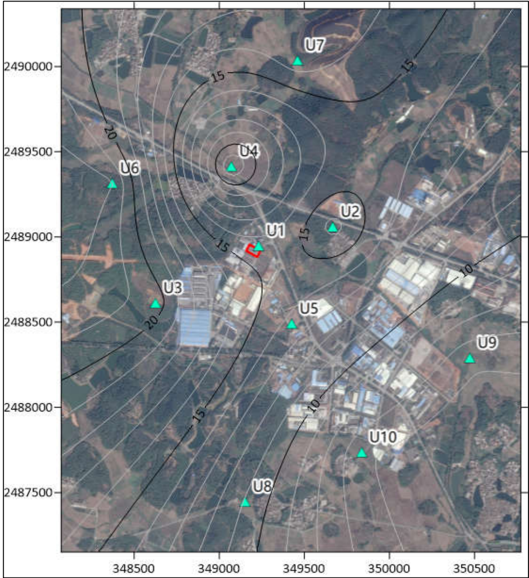
图 4.2.2-2 地下水水位等高线图
