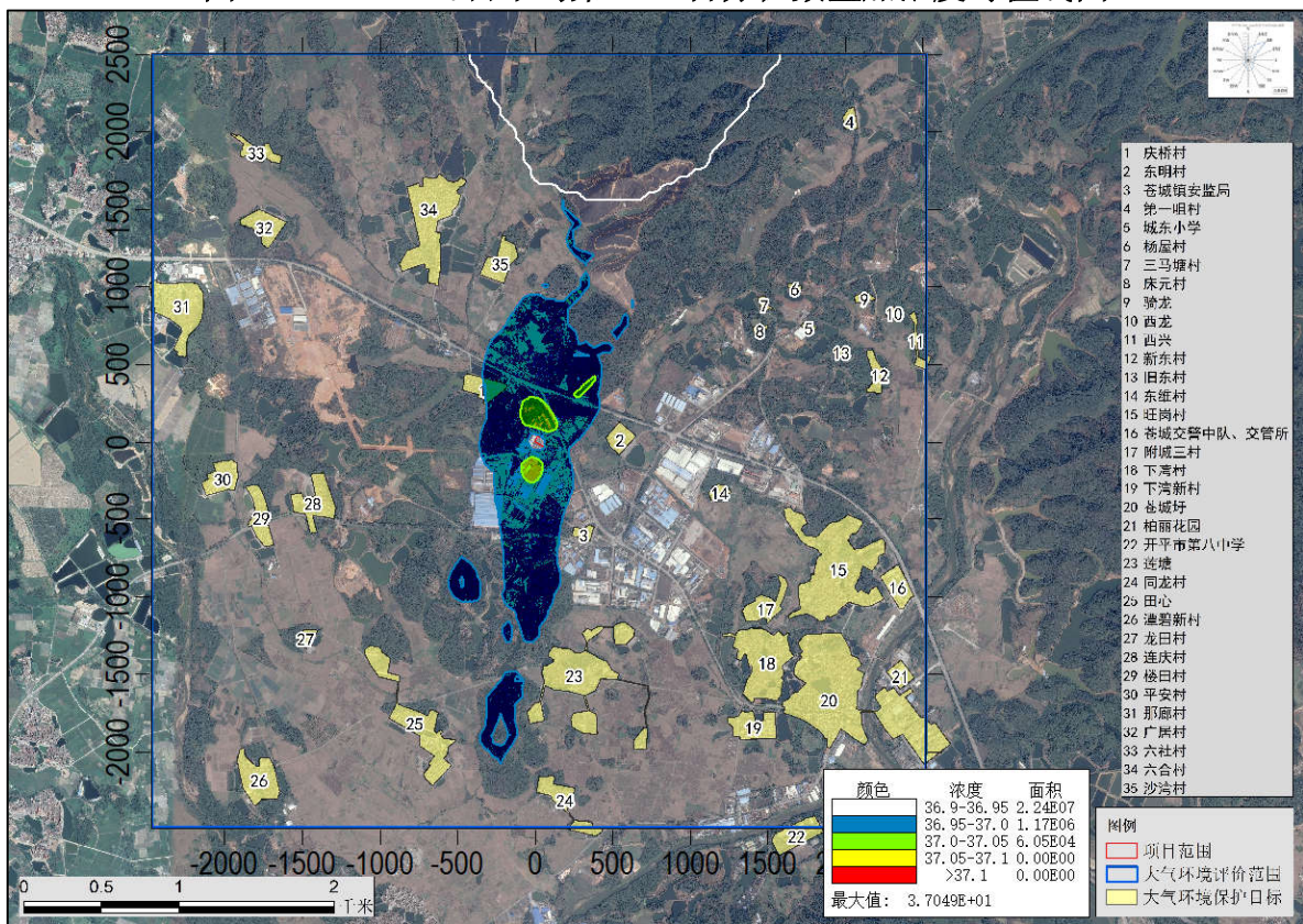
图 5.2.3-35 PM 10 年平均叠加浓度等值线图
