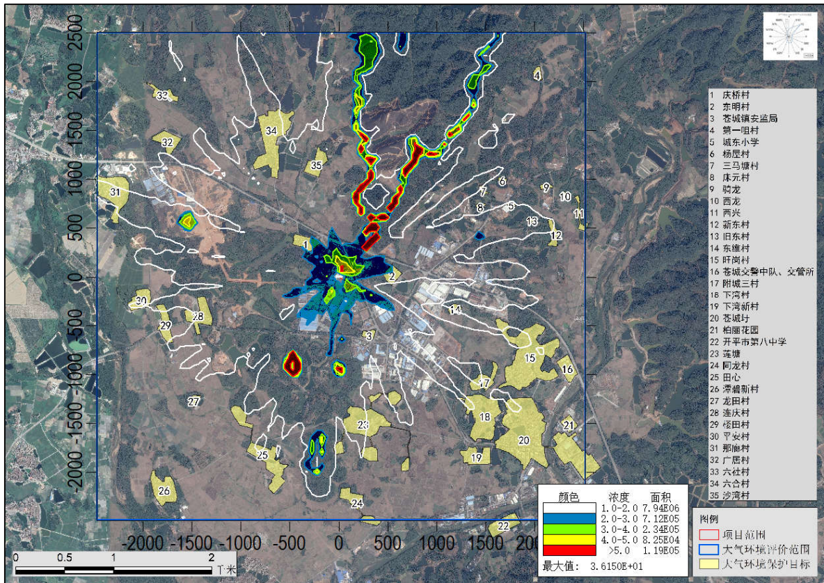
图 5.2.3-17 \text{SO}_2 1h 平均浓度最大贡献值等值线图
