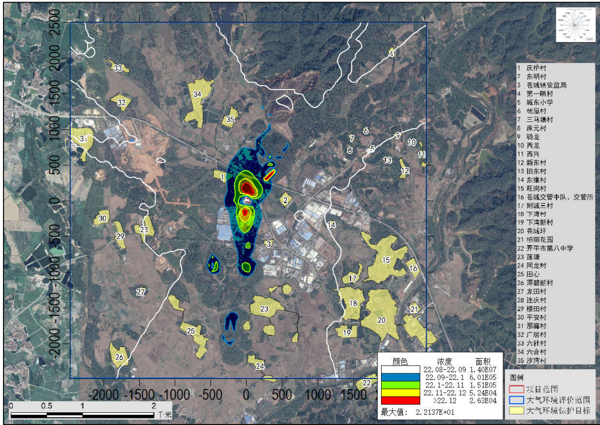
图 5.2.3-37 PM 2.5 年平均叠加浓度等值线图
