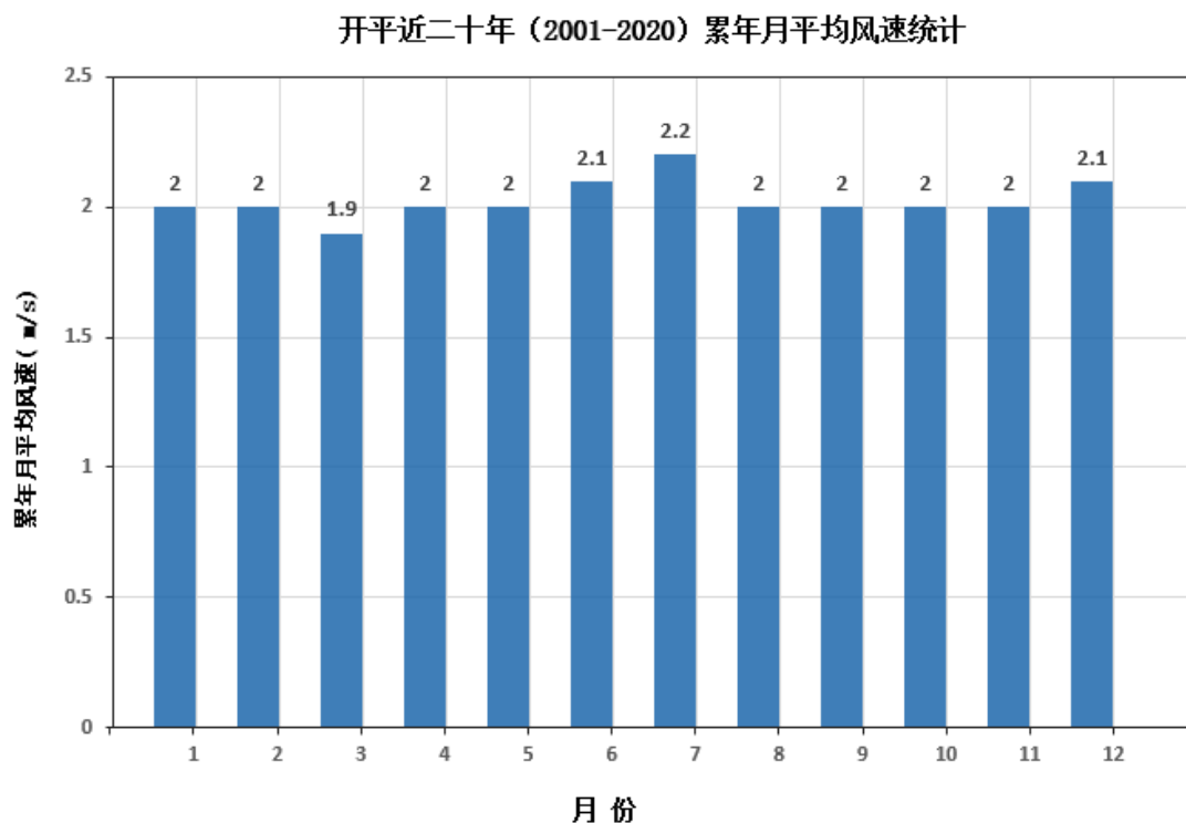
图 5.2.3-1 开平近 20 年月平均风速统计情况（单位: °C）
