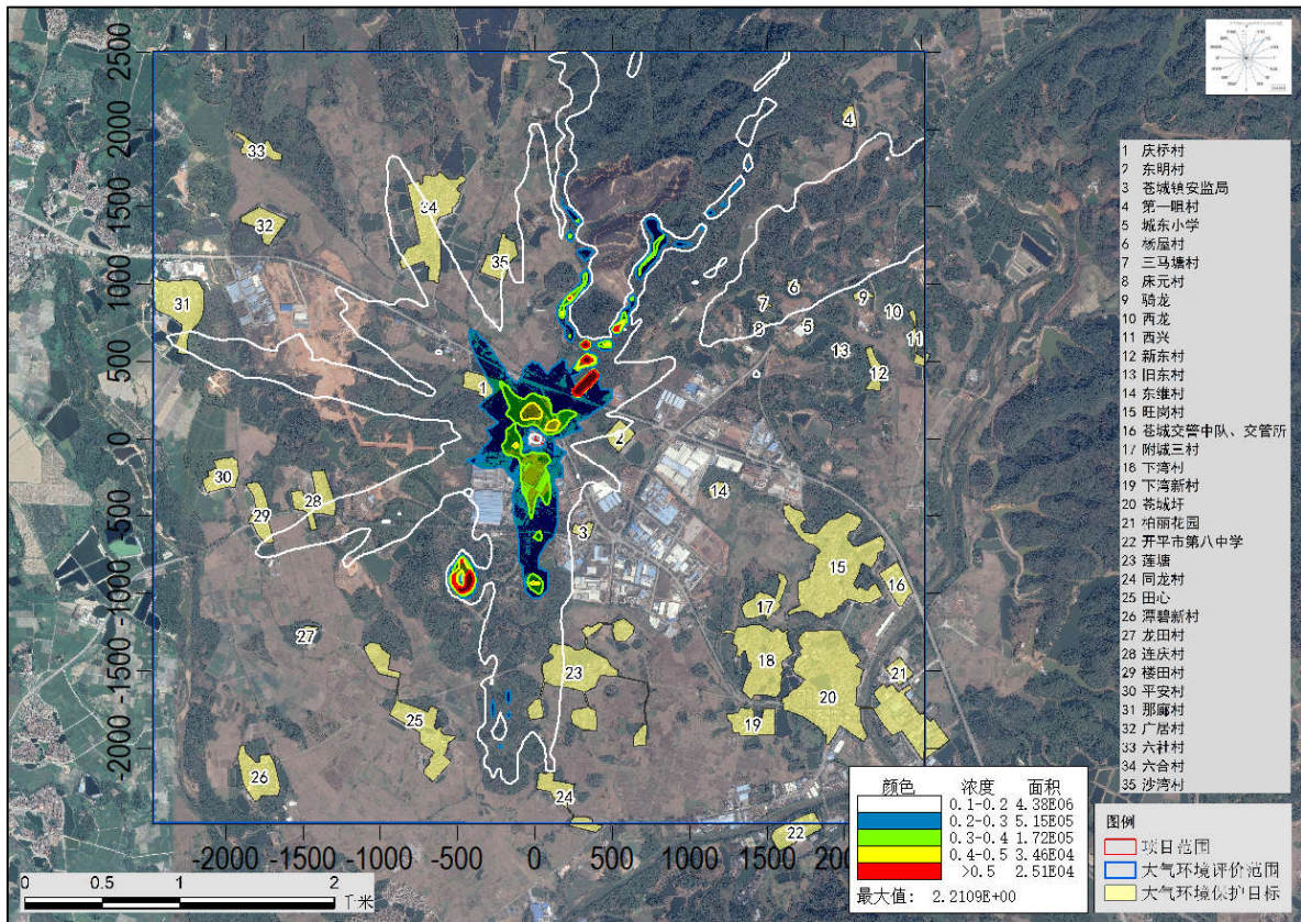
图 5.2.3-18 \text{SO}_2 日平均浓度最大贡献值等值线图
