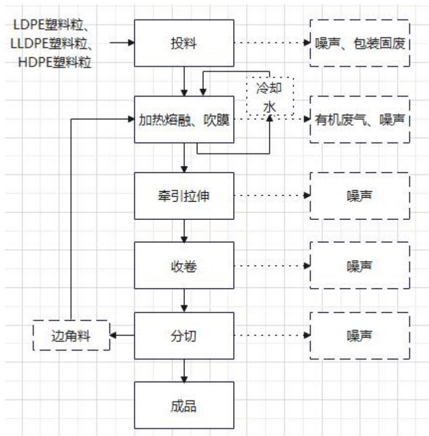
图 2-2 热收缩膜、缠绕膜生产工艺及产污流程图
