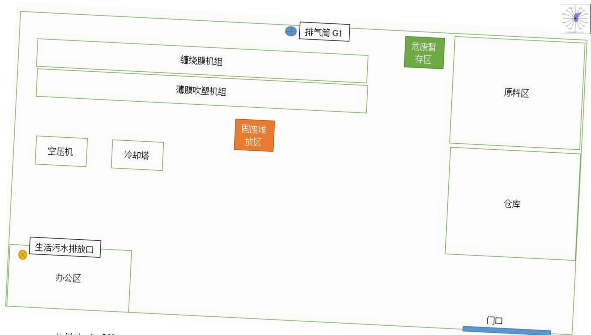
附图四 项目总平面布置图
