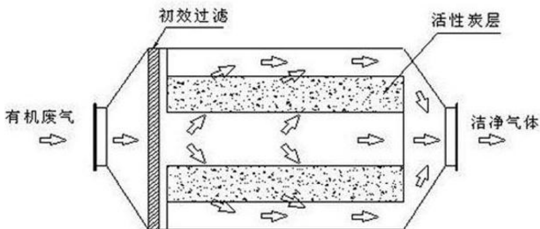
图 4-2 单极活性炭工作原理图
