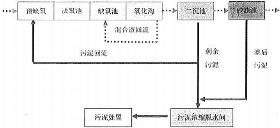
荷塘污水处理厂处理工艺流程图
