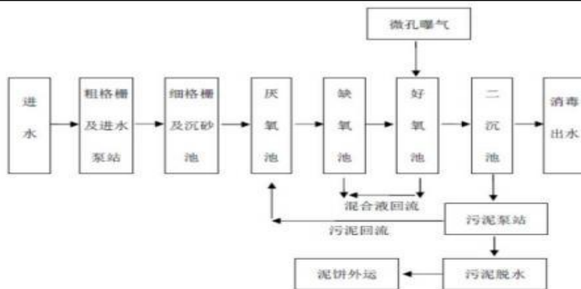
图 4-1 荷塘镇污水处理厂一、二期工程工艺流程图
