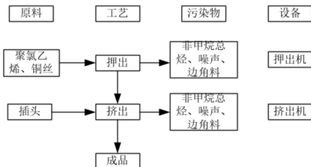
图 2-3 插头线生产工艺流程及产污环节示意图
