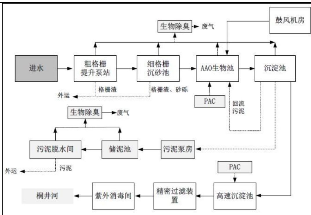
图 4-3 棠下污水处理厂二期工程废水处理工艺流程图
