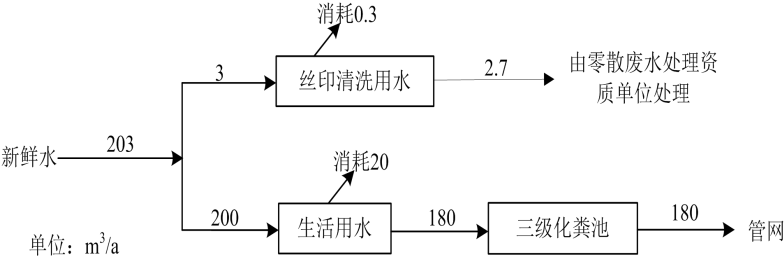
图 2-1 水平衡图
