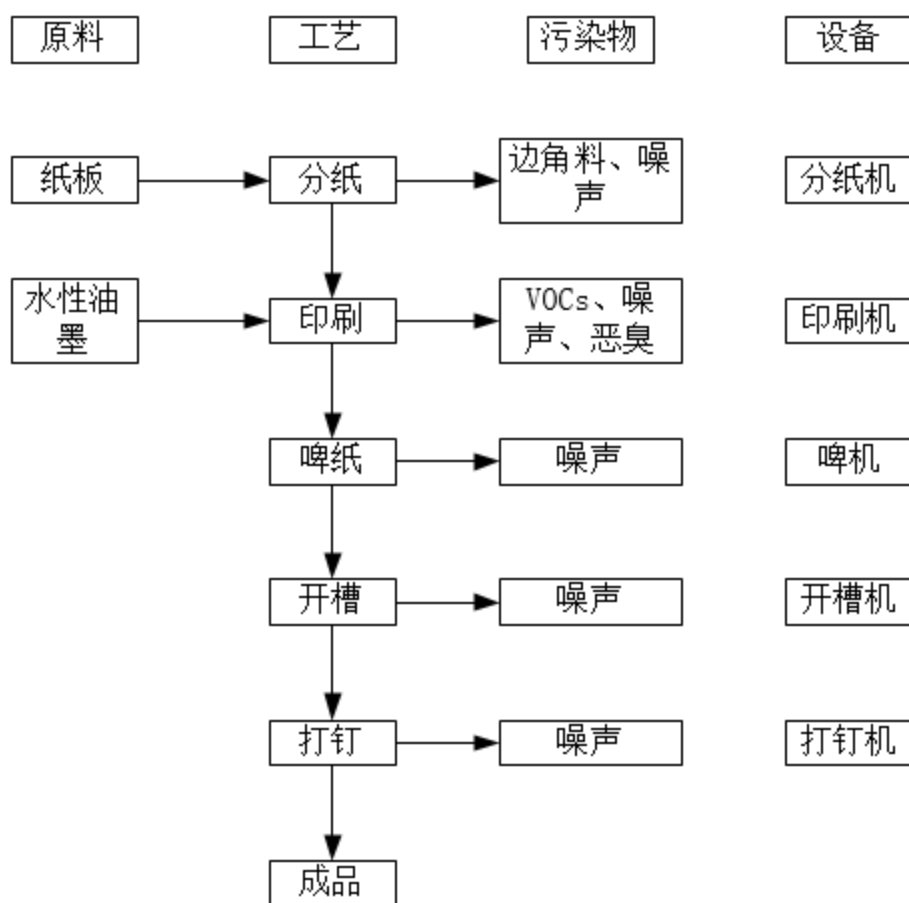
图 2-2 纸箱生产工艺流程及产污环节示意图
