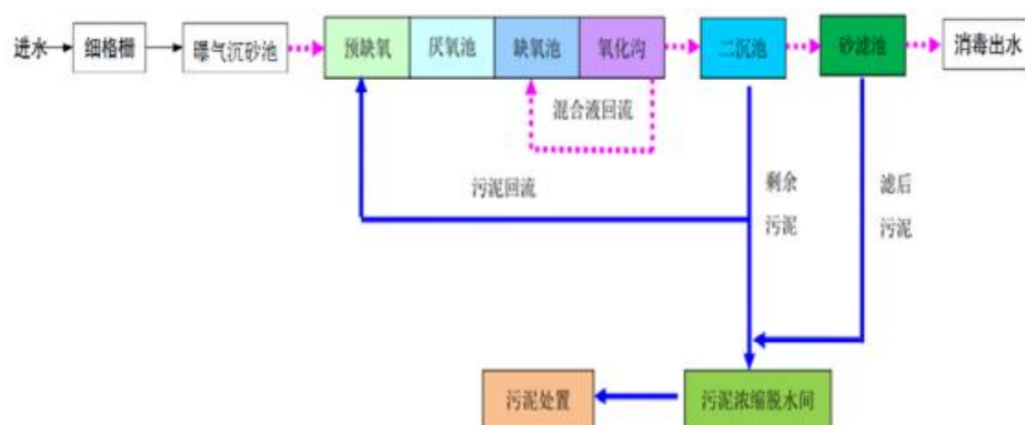
图3. 荷塘镇生活污水处理厂工艺流程图
