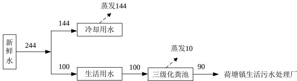
图1. 项目水平衡图（单位：m 3 /a）
