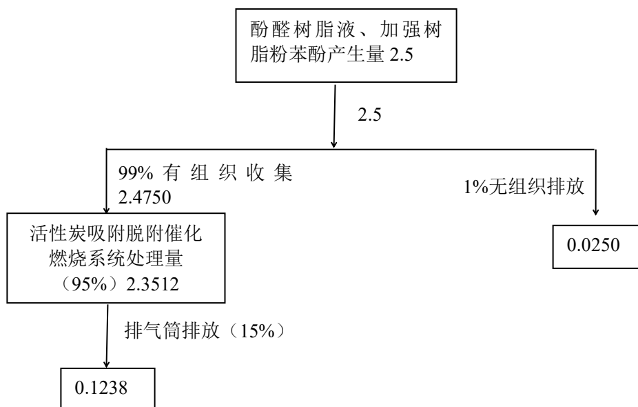
图2-2 苯酚平衡图（单位：t/a）
