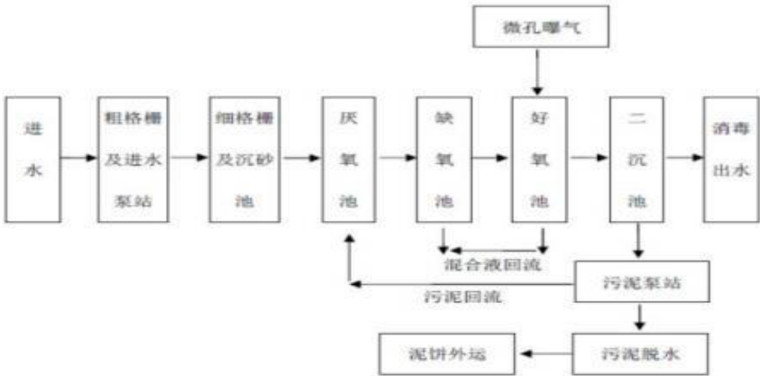
图 4-12.2 荷塘镇污水处理厂一、二期工程工艺流程图
