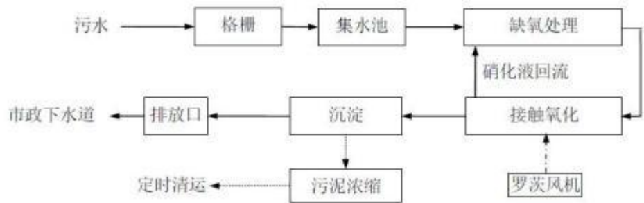
图 4-12.1 一体化污水处理设施工艺流程图
