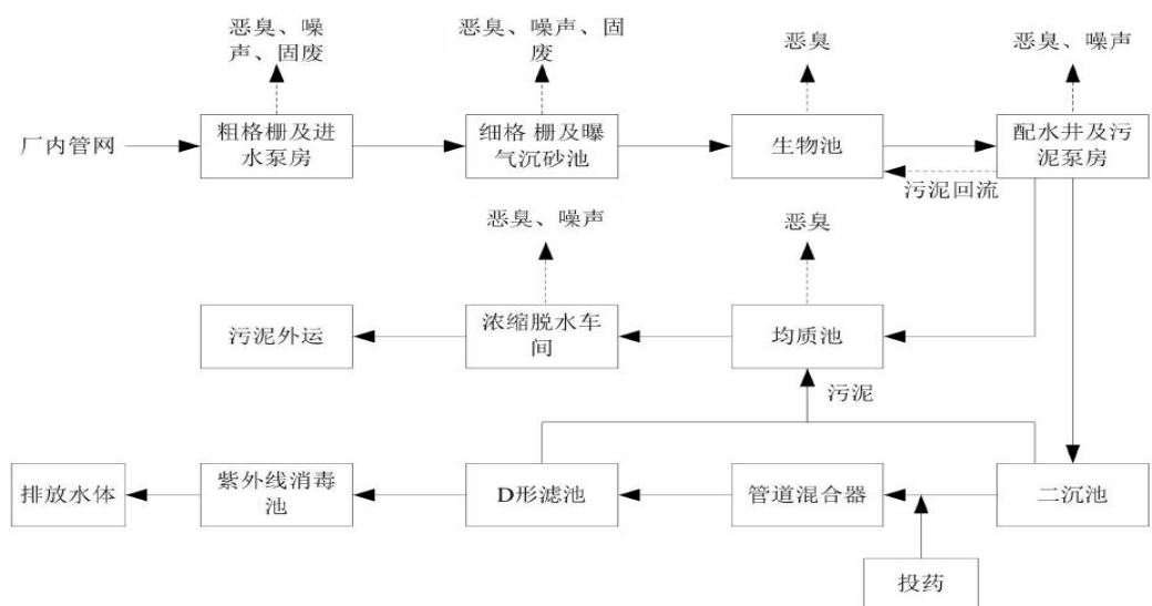
图4-1 杜阮污水处理厂污水处理工艺流程图
