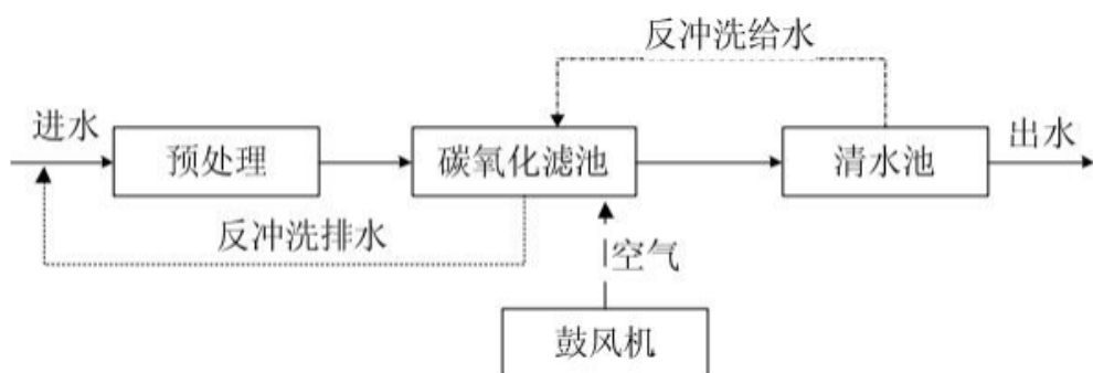
图 3.2-7 碳氧化滤池工艺流程图
