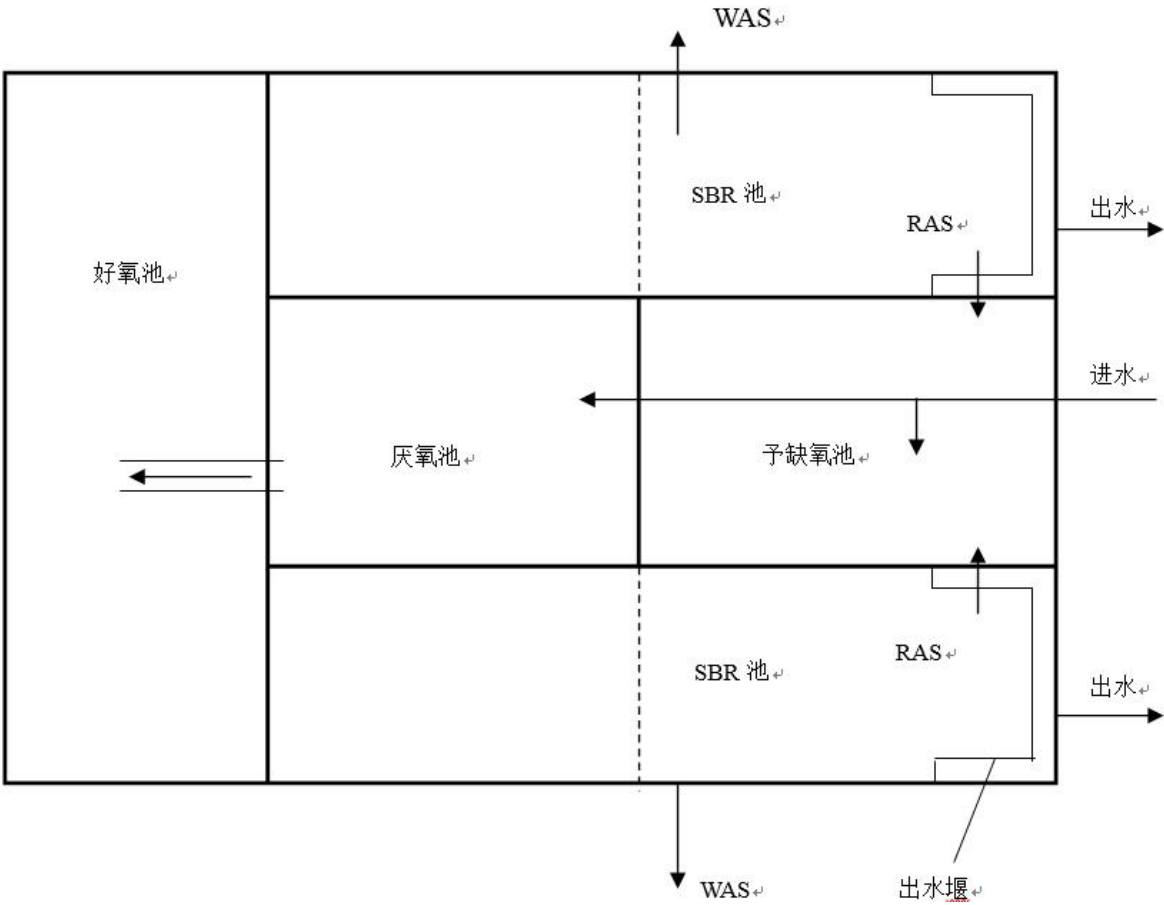
图 3.2-4 MSBR 系统原理图
