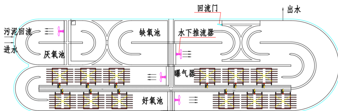
图 3.2-6 AAO 氧化沟系统原理图
