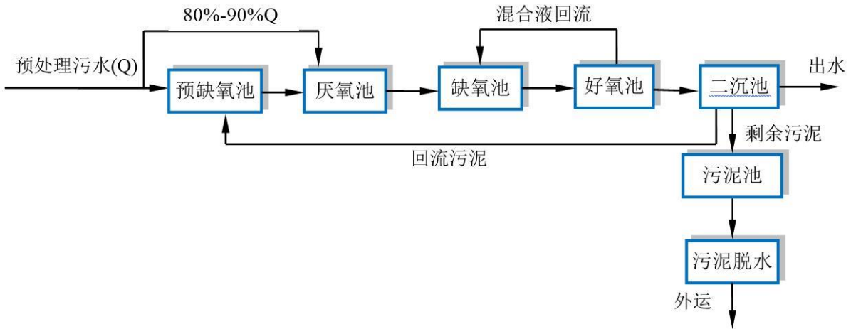
图 3.2-3 改良 AAO 工艺基本流程图
