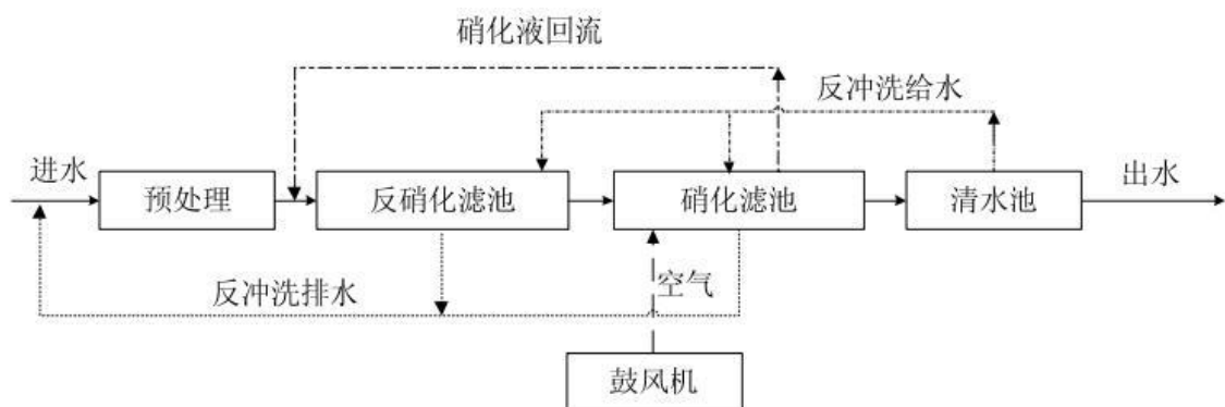
图 3.2-9 前置反硝化滤池+硝化滤池两级组合工艺流程图
