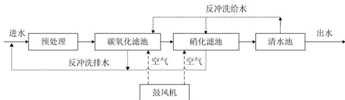
图 3.2-8 碳氧化滤池+硝化滤池两级组合工艺流程图
