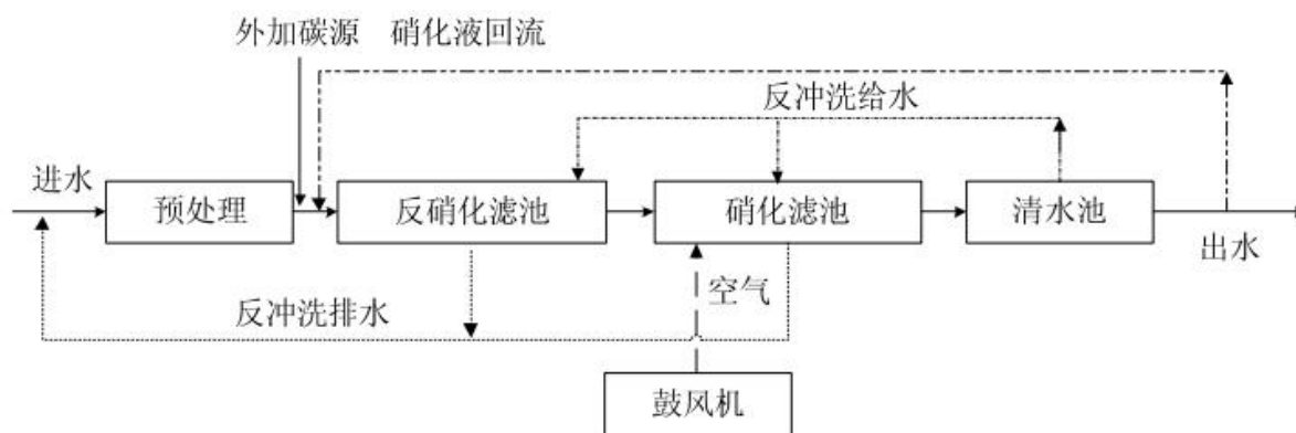
图 3.2-11 外加碳源前置反硝化滤池两级组合工艺流程
