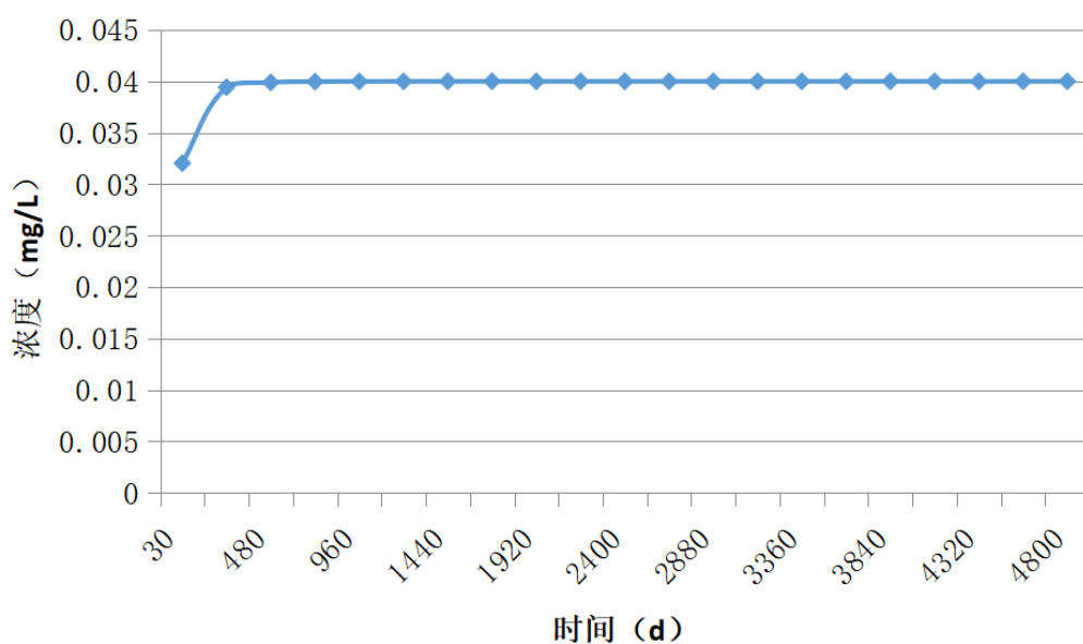
图 5.3-2 非正常工况下废水泄漏后迁移距离及浓度变化曲线图 (COD)
