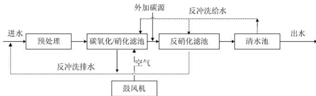
图 3.2-10 外加碳源后置反硝化滤池两级组合工艺流程图
