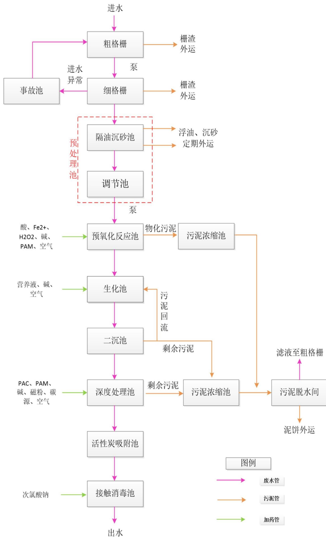
图 6.2-1 污水处理工程工艺流程图
