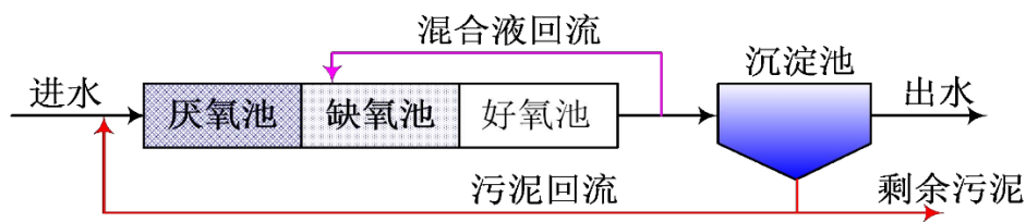
图 3.2-2 AAO 工艺基本流程
