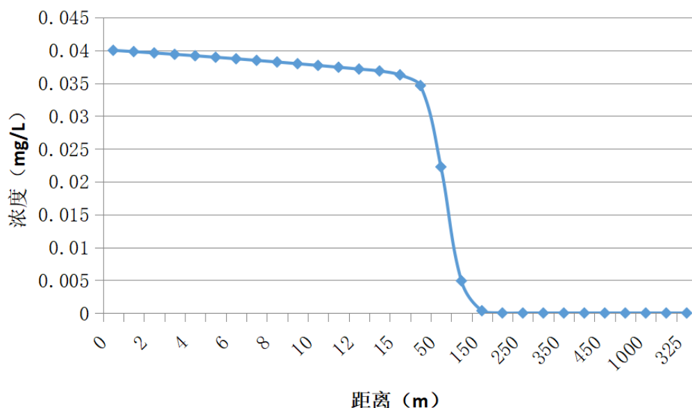
图 5.3-3 非正常工况下废水泄漏后时间及浓度变化曲线图 (COD)
