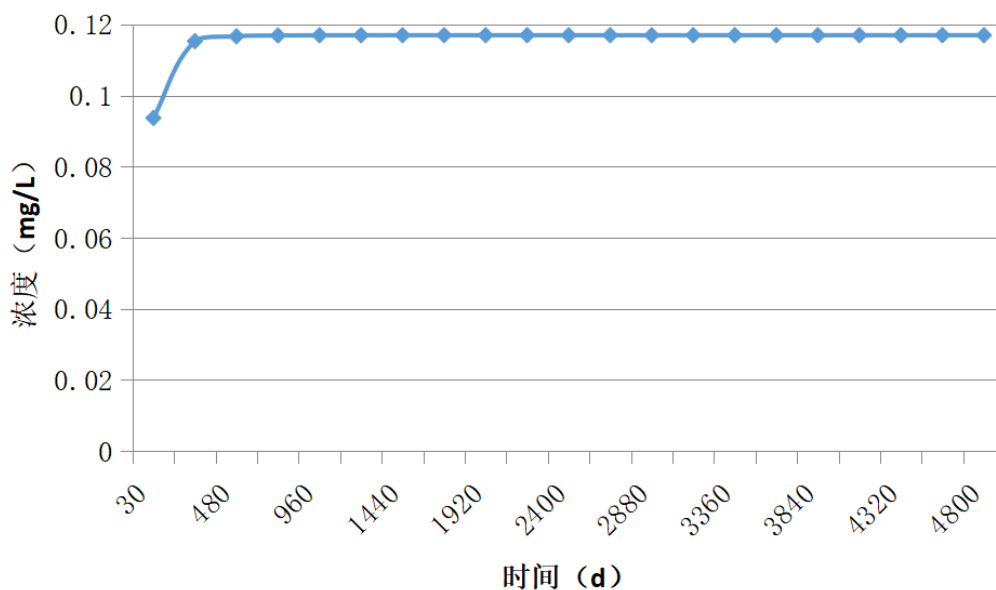
图 5.3-1 非正常工况下废水泄漏后时间及浓度变化曲线图 (COD)
