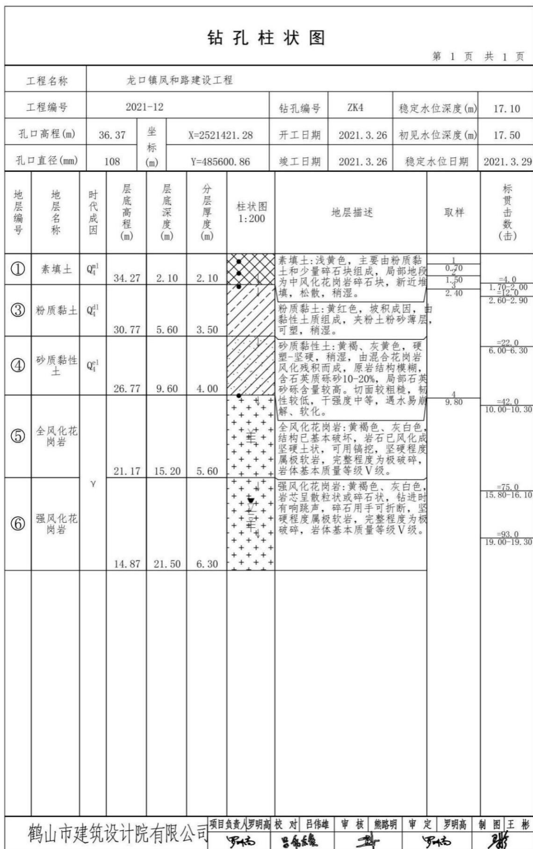
图 4.5-2 规划区钻孔柱状图 (4)
