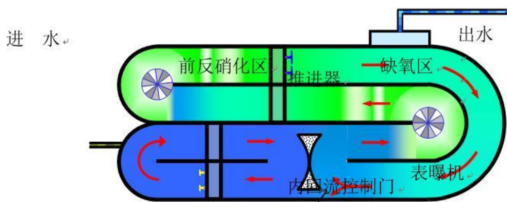
图 3.2-5 Carrousel2000 型工艺原理
