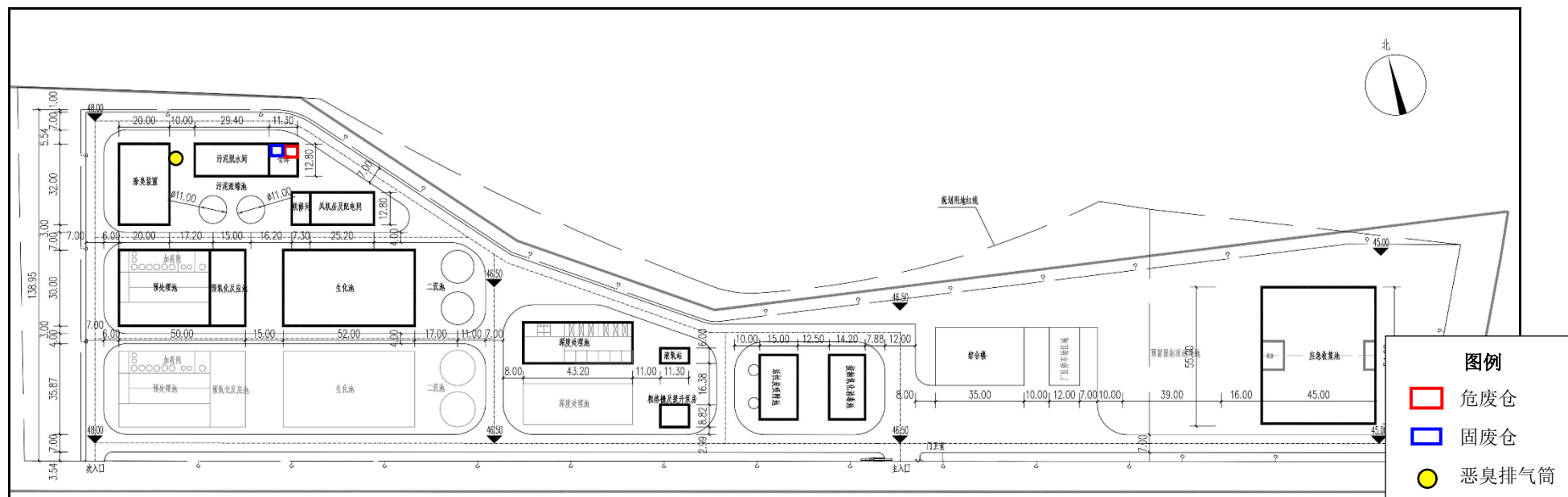
图 3.1-4 项目污水处理工程平面布置图
