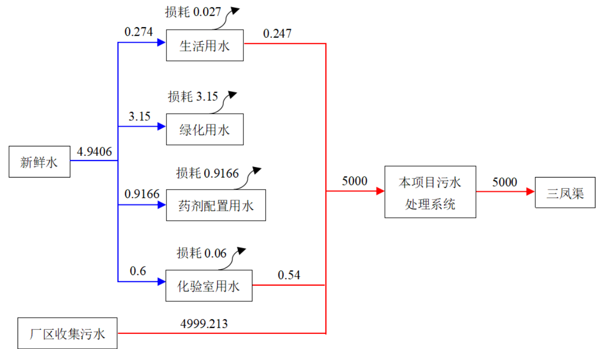
图 3.1-5 项目晴天用水一览表 单位：m³/d
