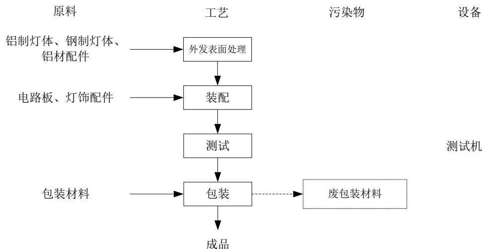
图5. 成品生产工艺流程图
