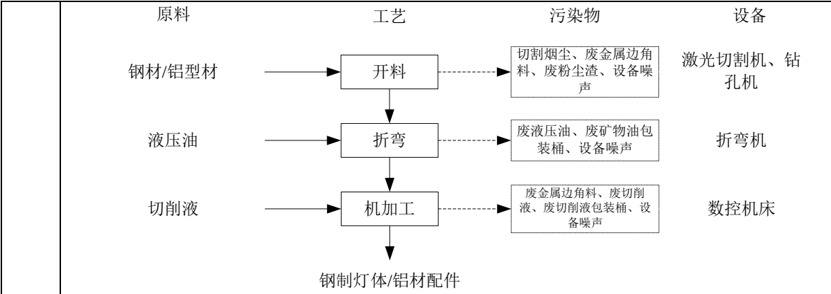
图3. 钢制灯体/铝材配件生产工艺流程图
