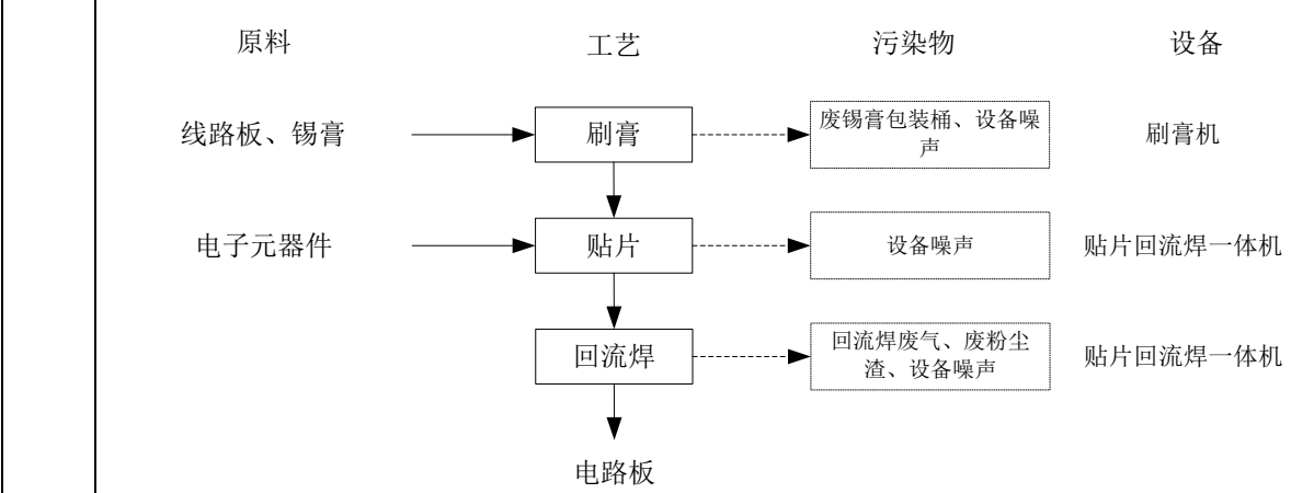
图4. 电路板生产工艺流程图
