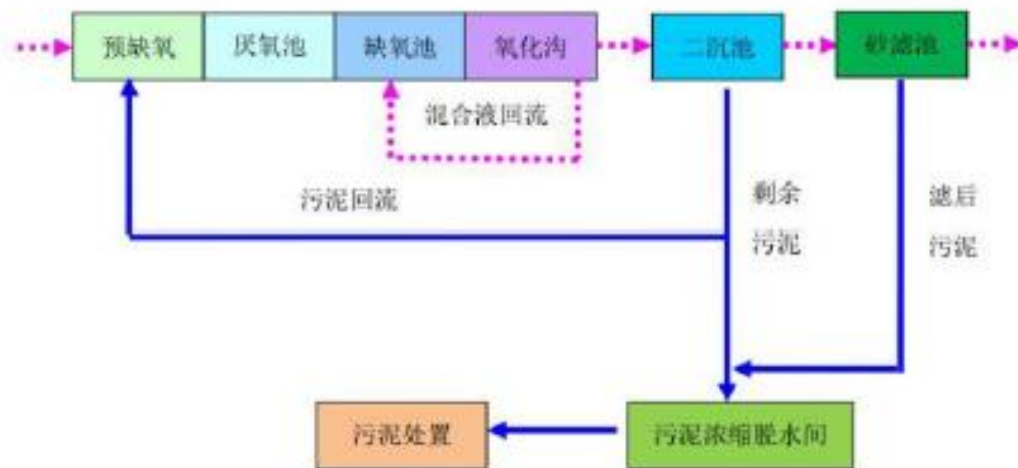
图6. 荷塘镇污水处理厂处理工艺流程图
