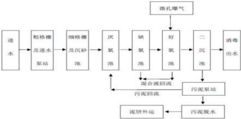
图 4-2 荷塘镇污水处理厂一、二期工程工艺流程图
