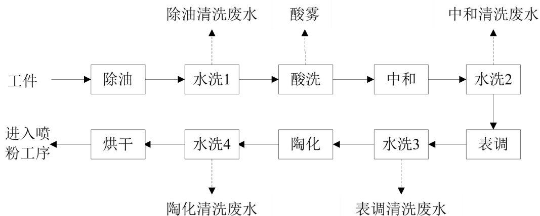
图2-3 前处理生产线生产工艺流程及产污环节图
