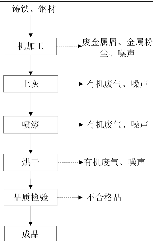
图2-2 机床零配件、民用航天器零配件生产工艺流程及产污环节图
