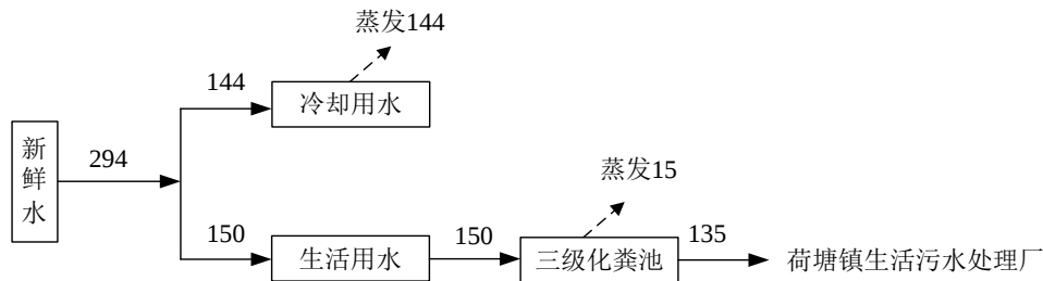
图1. 项目水平衡图（单位：m 3 /a）
