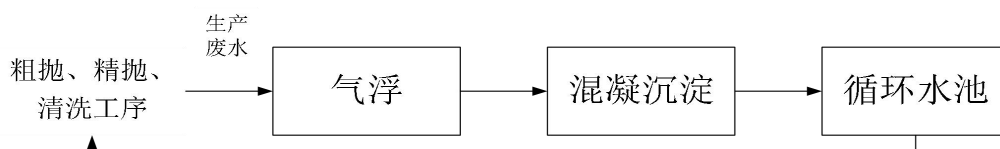
图 3 生产废水回用流程图
