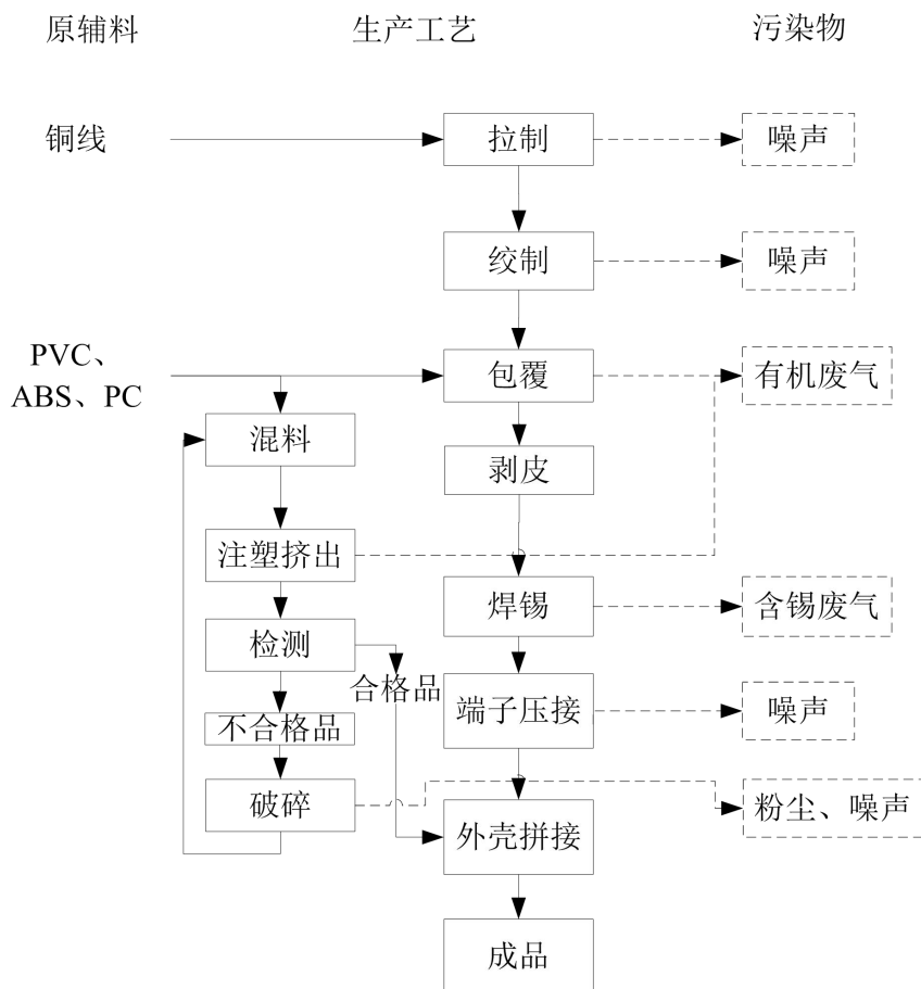
图 2-1 工艺流程图
