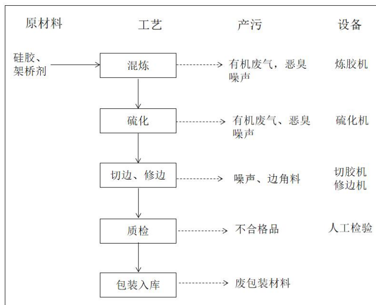
图 2-2 硅胶制品生产工艺流程图
