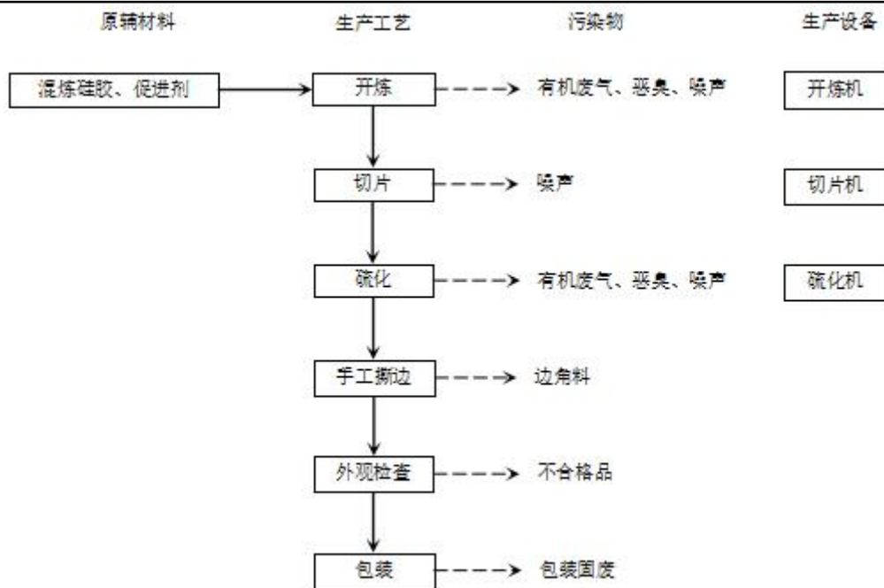
图2-3 生产工艺流程图
