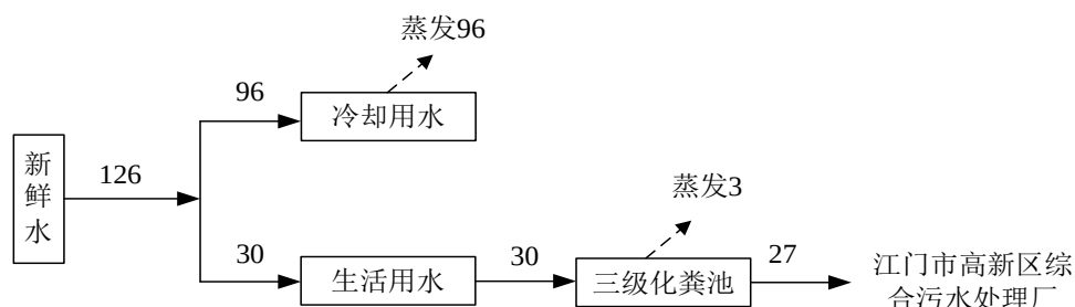
图1. 项目水平衡图（单位： \text{m}^3/\text{a} ）
