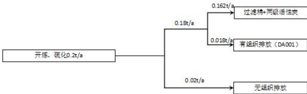
图 2-1 项目 VOC 平衡图 (t/a)
