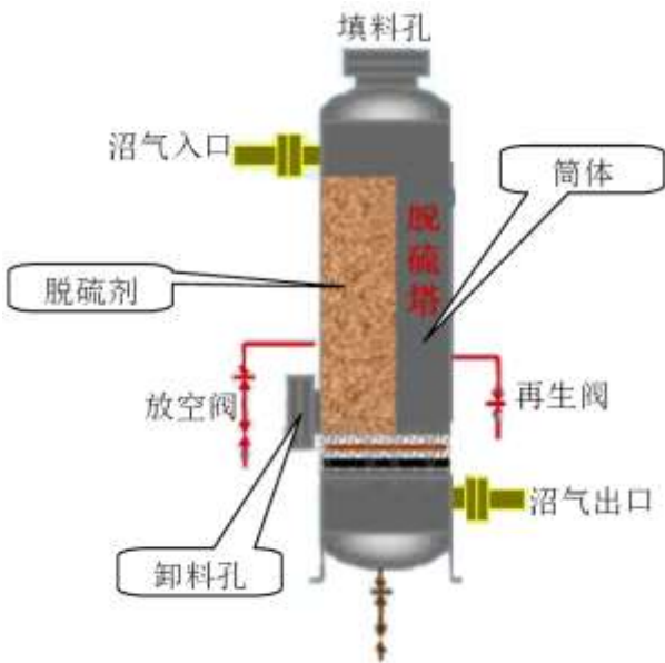
图 7.3-3 脱硫塔结构图
