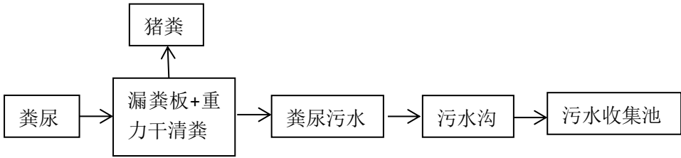
图 4.2-2 项目清粪工艺流程图
