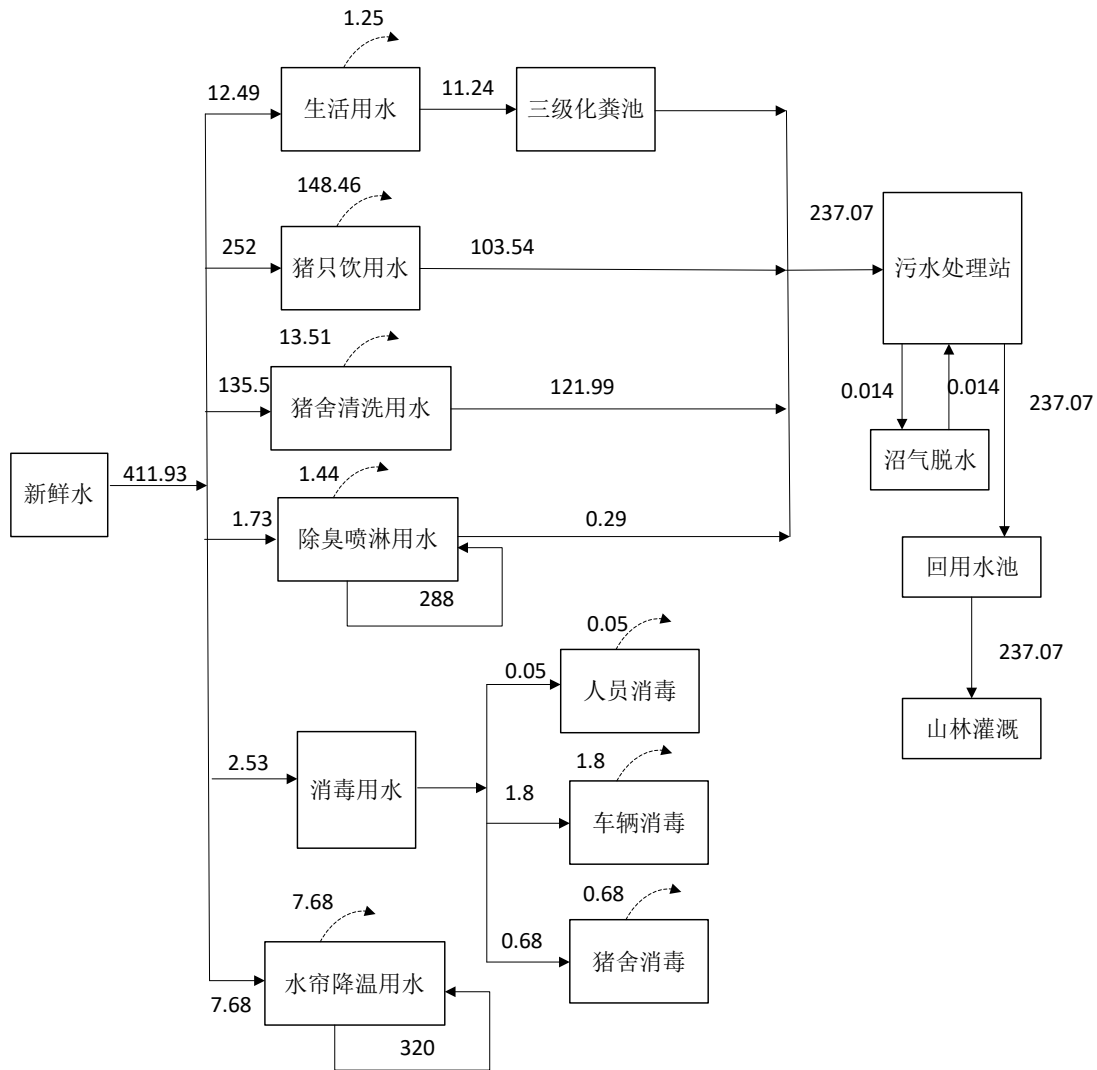
图 4.1-2 项目水平衡图 (m³/d, 夏季, 非雨天)
