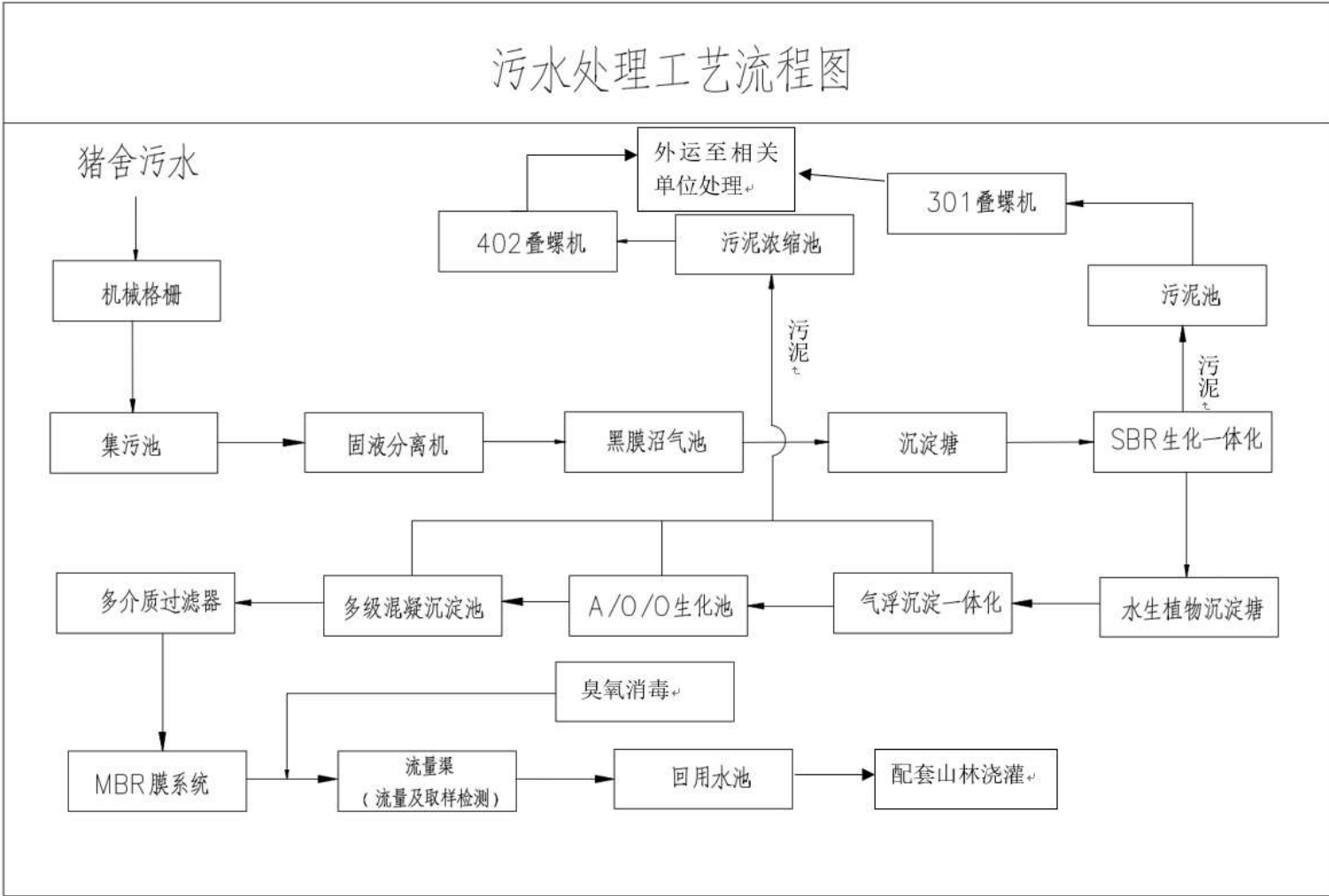
图 4.2-9 项目废水处理工艺流程图
