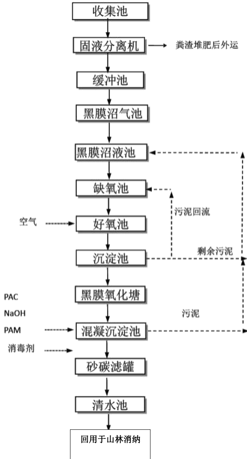
图 3.2-10 项目废水处理工艺流程图
