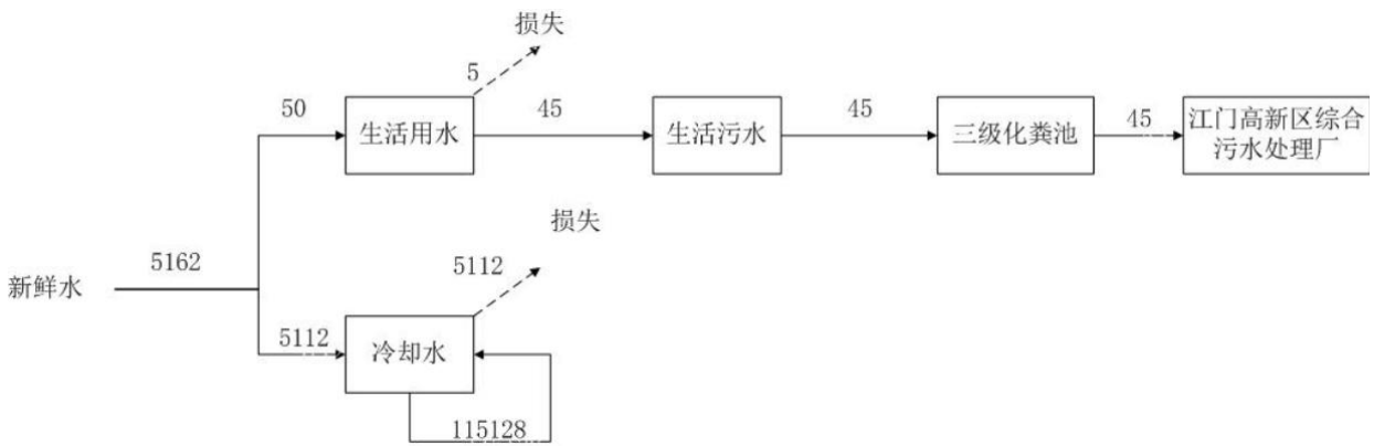
图 2-1 远期水平衡图 (单位: \text{m}^3/\text{a} )
