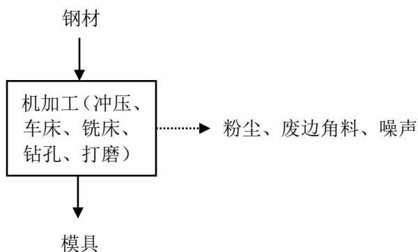
图 2-3 模具生产流程图
