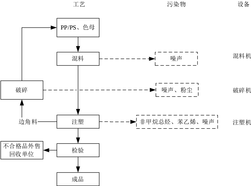
图2. 生产工艺流程图
