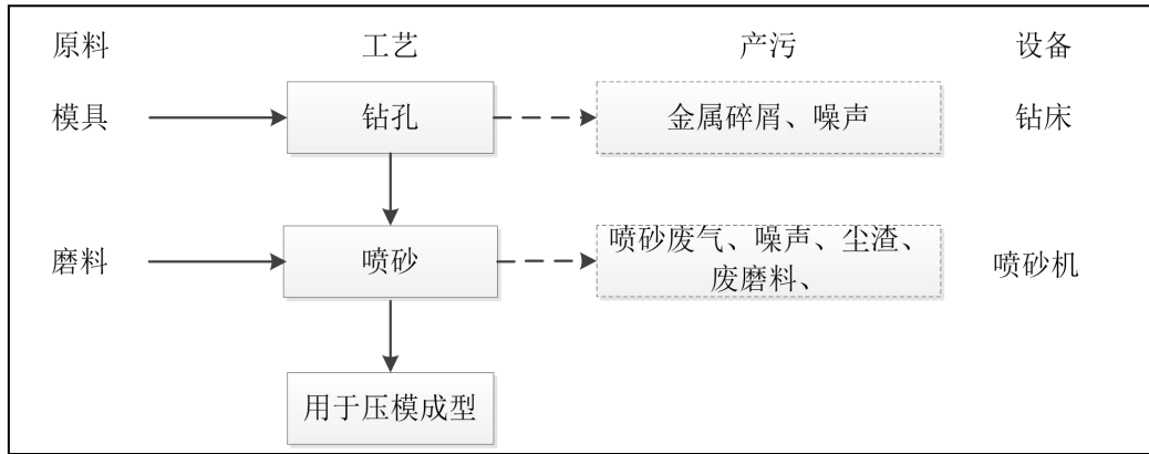
图 2-2 模具维修工艺流程图
