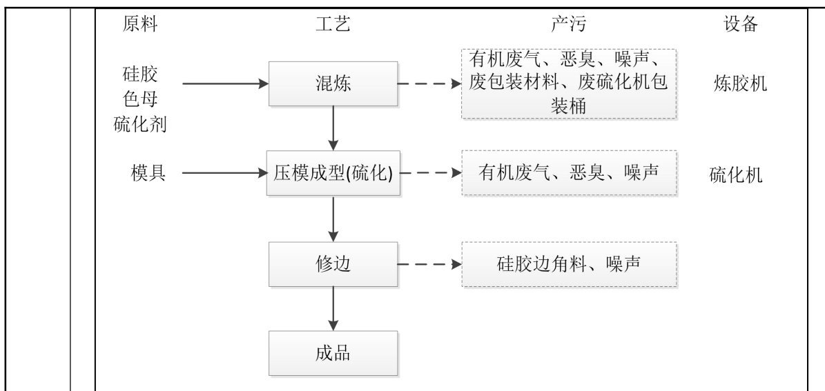
图 2-2 硅胶密封圈生产工艺流程图
