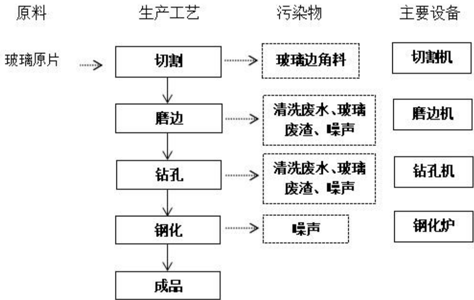
图 2-1 钢化玻璃生产工艺流程图
