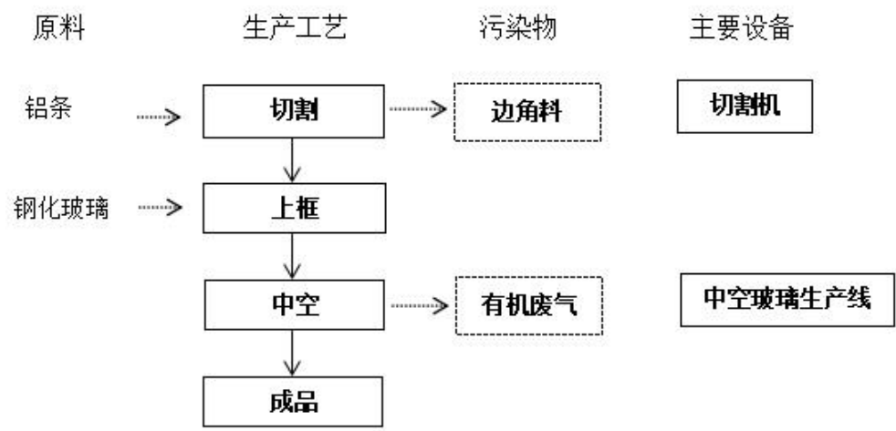
图 2-2 中空玻璃生产工艺流程图
