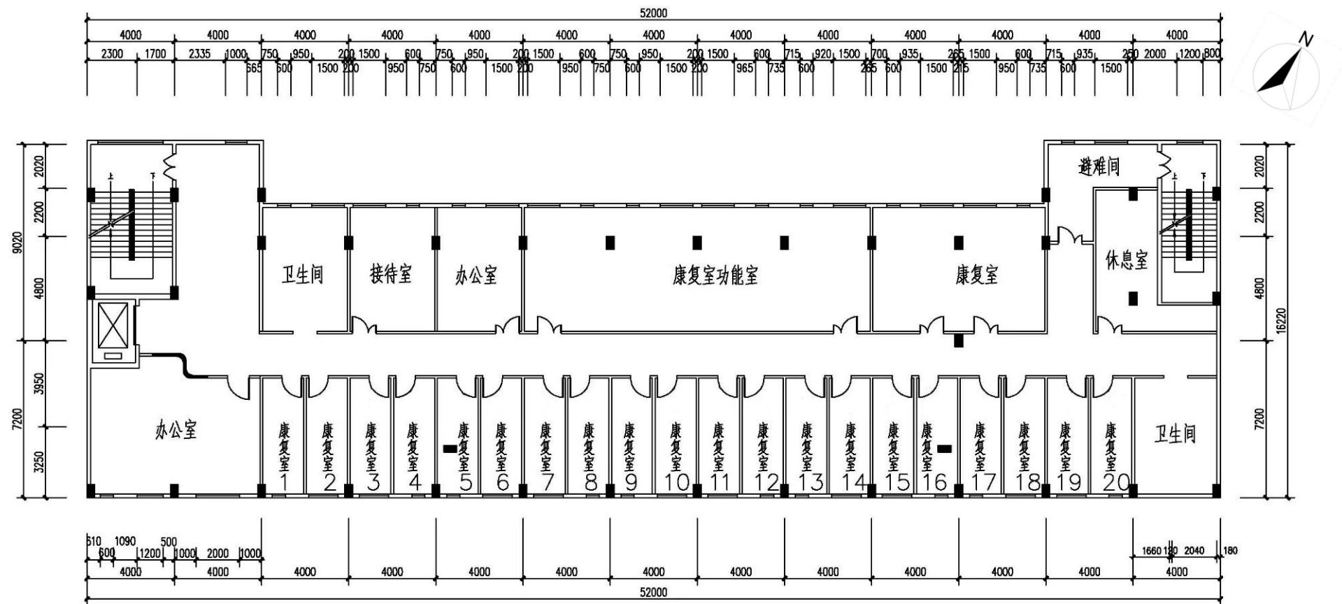
附图 8 医养综合大楼三层平面图
