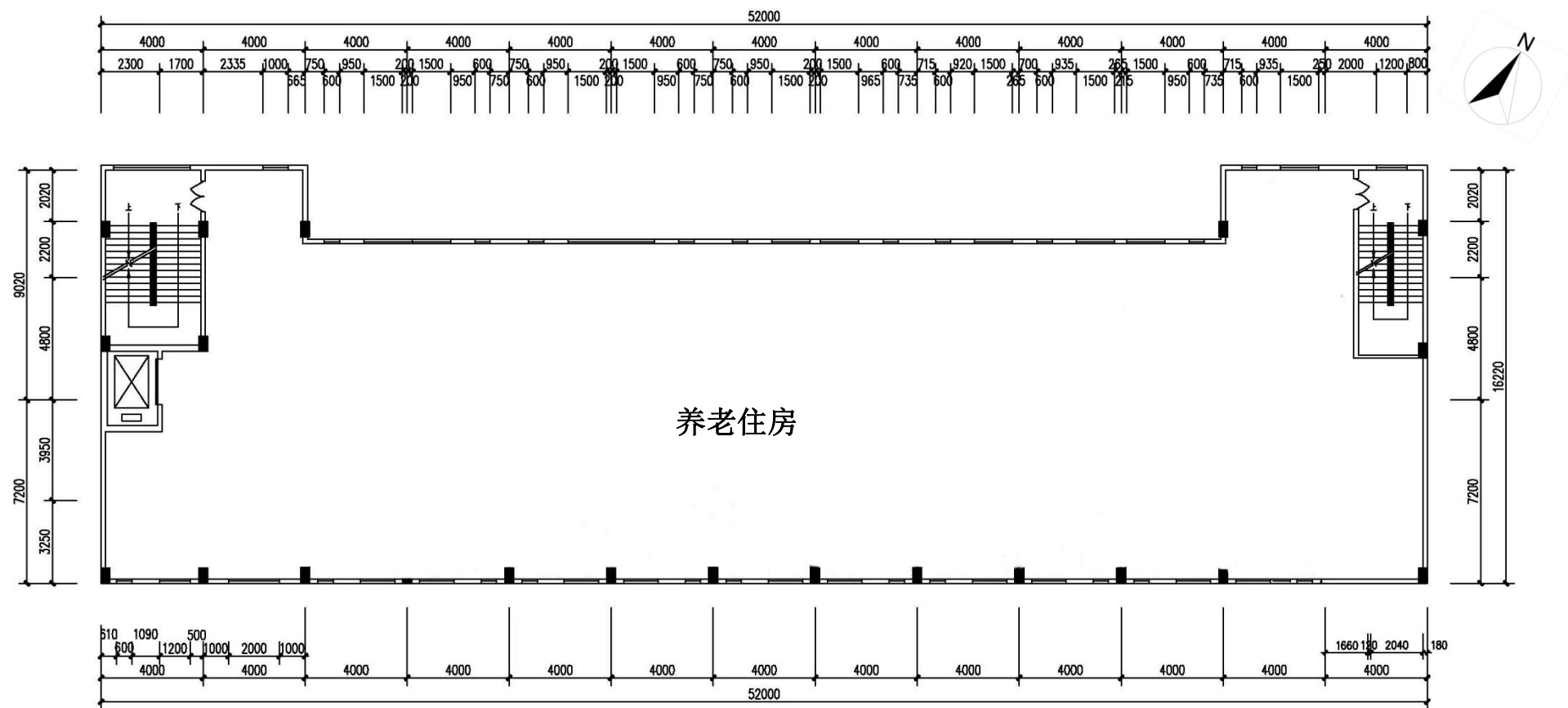
附图 10 医养综合大楼五层平面图
