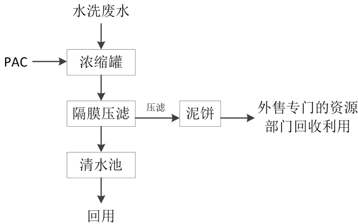
图 4-2 生产废水处理工艺流程图
