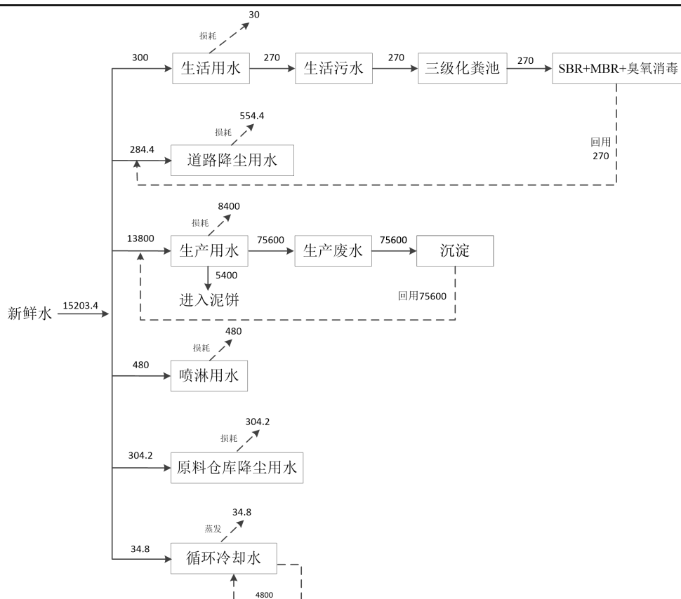
图 2-2 水平衡图 单位: m³/a
