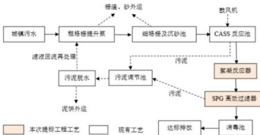
图 7. 开平市水口污水处理厂处理工艺流程图
