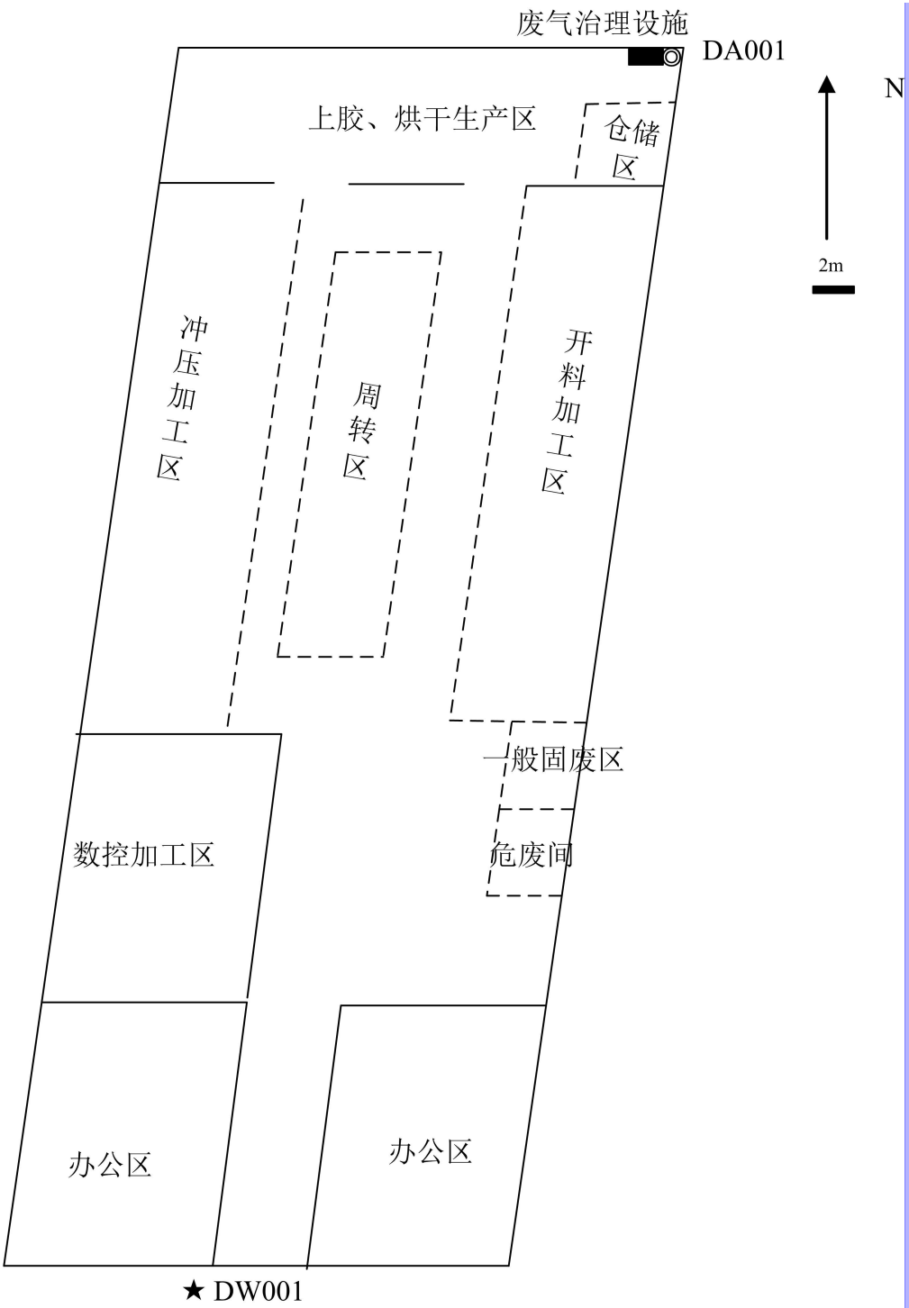
附图 3. 平面布置图
