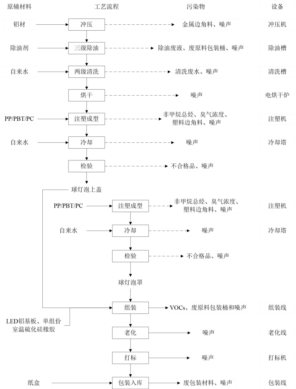
图 2-5 LED 球灯泡生产工艺流程及产污环节图
