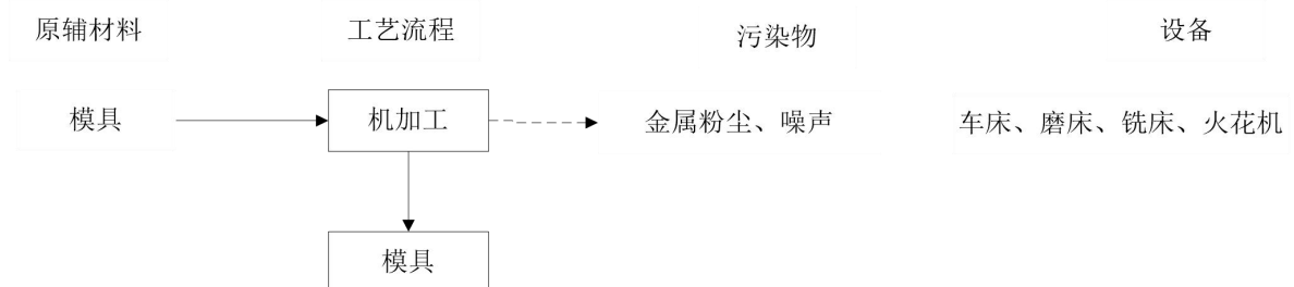
图 2-6 模具维修工艺流程
