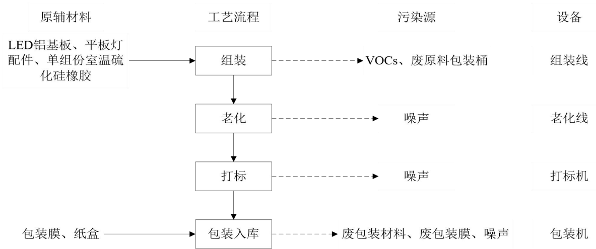
图 2-4 平板灯生产工艺流程及产污环节图
