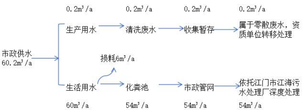
图 2-1 水量平衡图
