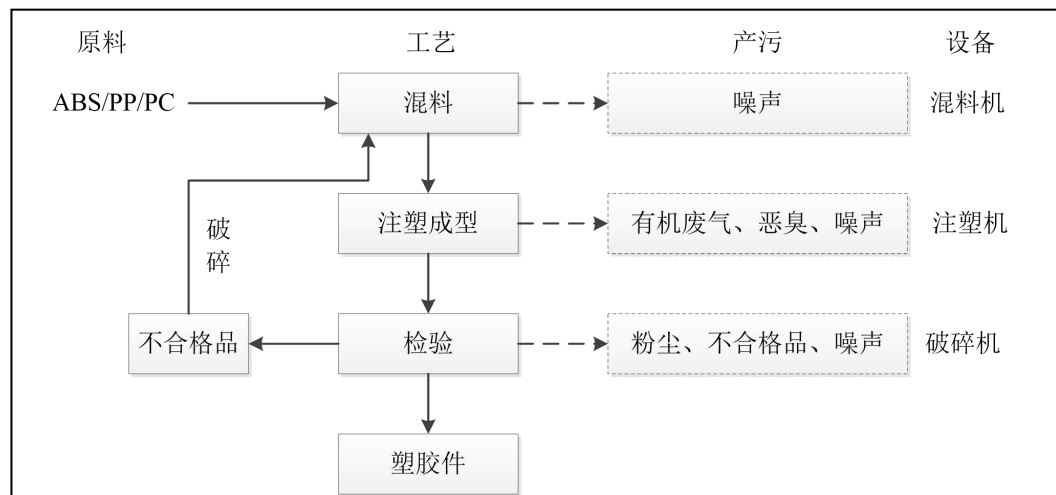
图 2-3 塑胶件生产工艺流程图
