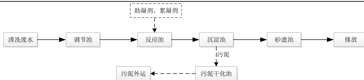
图4-1 废水处理工艺流程图
