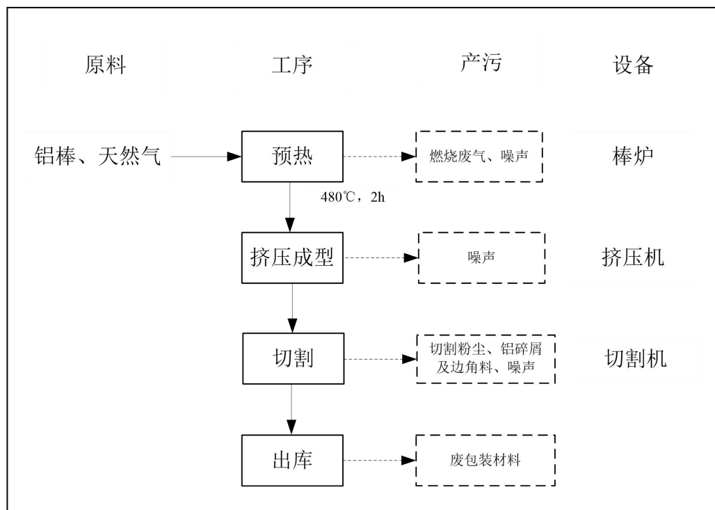
图 2-1 铝型材工艺流程图
