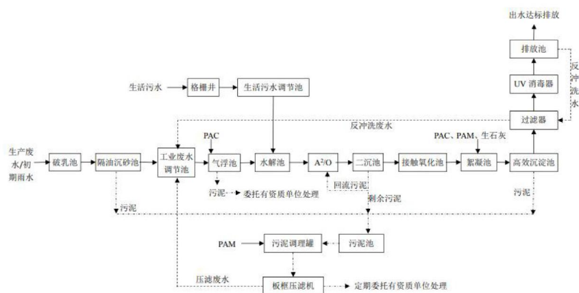
图 4. 龙胜镇汽配产业园污水处理厂处理工艺流程图
