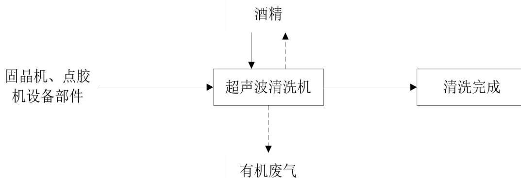
图 2-2 设备部件清洗工艺流程及产污环节图
