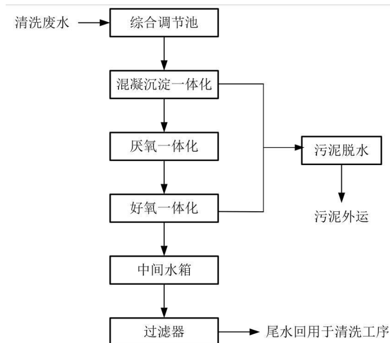
图 5. 废水处理工艺图
