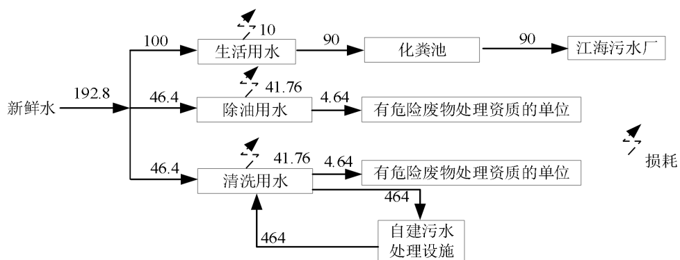
图 1. 扩建项目水平衡图 (t/a)
