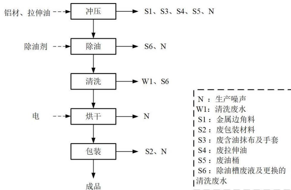
图 2. 生产工艺流程图
